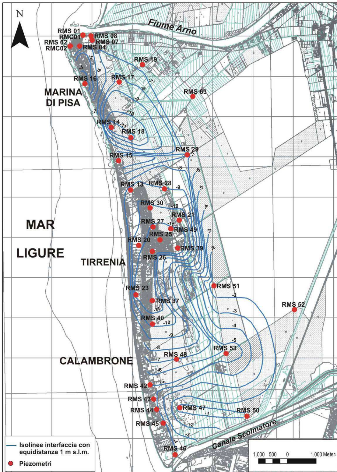
Fig. 38 - Carta della posizione dell'interfaccia acqua dolce-acqua salata nella falda freatica per il mese di aprile 2009 nell'area compresa tra il Fiume Arno e il canale Scolmatore.
