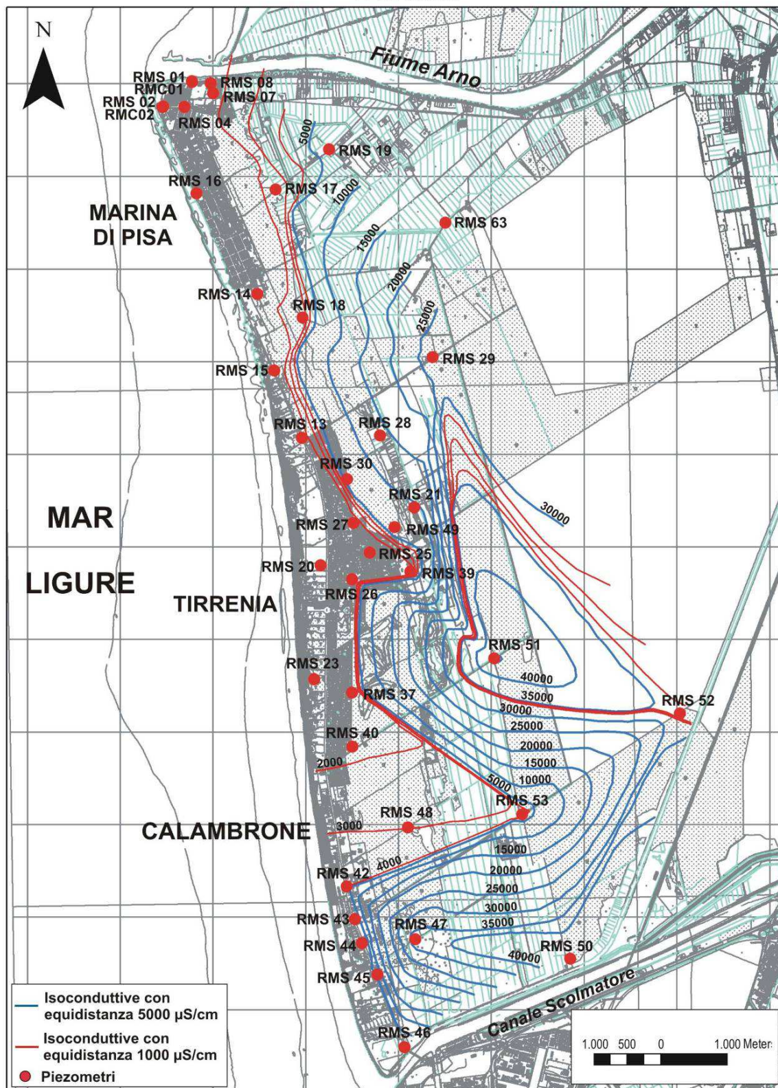
Fig. 34 - Carta delle isoconduttive della falda freatica riferite alla quota di -2,0 m s.l.m. per il mese di aprile 2009 nell'area compresa tra il Fiume Arno e il canale Scolmatore.
