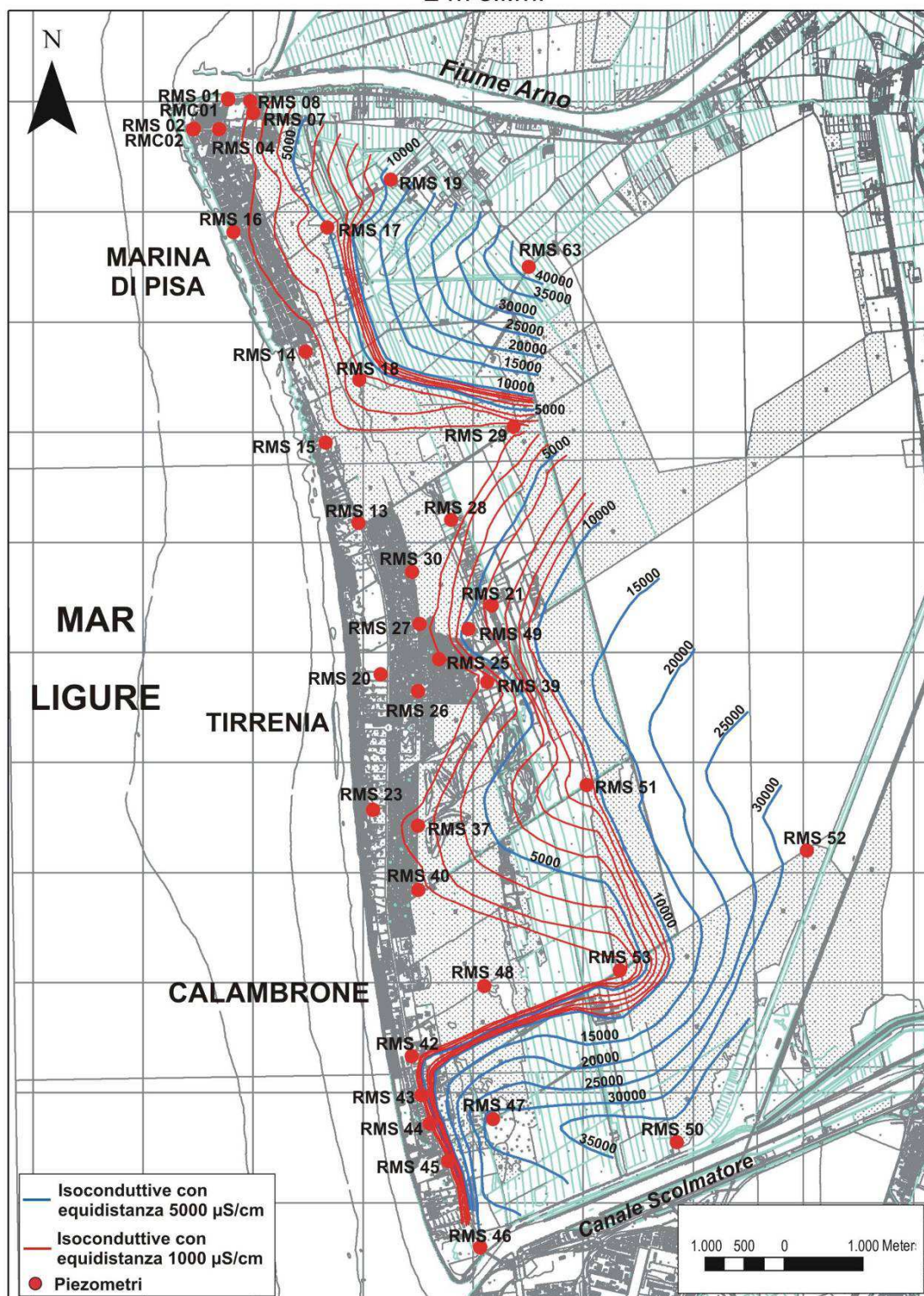
Fig. 36 - Carta delle isoconduttive della falda freatica riferite alla quota di -2,0 m s.l.m. per il mese di settembre 2009 nell'area compresa tra il Fiume Arno e il canale Scolmatore.
