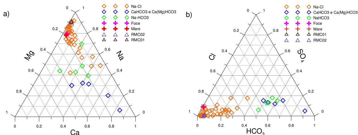
Fig. 41 - Diagrammi triangolari (a) Ca-Na-Mg e (b) \text{HCO}_3\text{-SO}_4\text{-Cl} per le acque dei piezometri superficiali, piezometri profondi (RMC01 e RMC02), foce del fiume Arno e acqua di mare.
