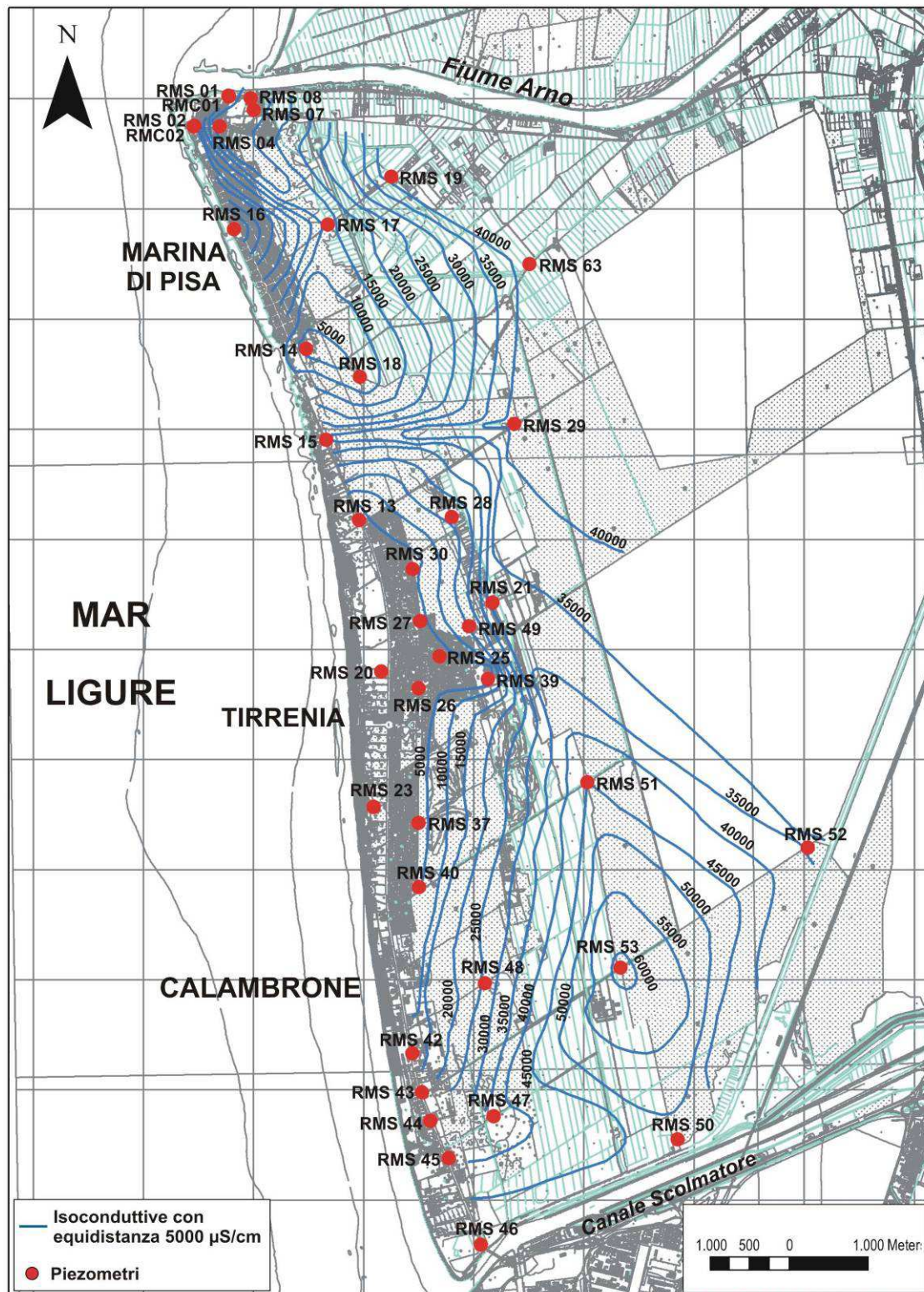
Fig. 37 - Carta delle isoconduttive della falda freatica riferite alla quota di -10,0 m s.l.m. per il mese di settembre 2009 nell'area compresa tra il Fiume Arno e il canale Scolmatore.
