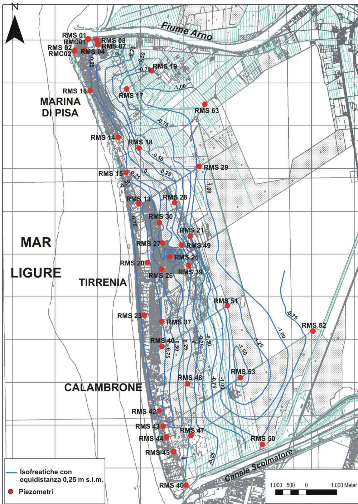
Fig. 30 - Carta delle isofreatiche dell'area compresa tra il Fiume Arno e il canale Scolmatore del mese di settembre 2009.
