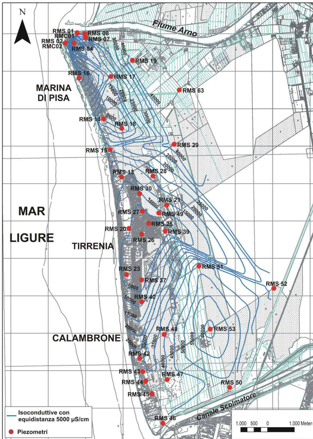
Fig. 35 - Carta delle isoconduttive della falda freatica riferite alla quota di -10,0 m s.l.m. per il mese di aprile 2009 nell'area compresa tra il Fiume Arno e il canale Scolmatore.
