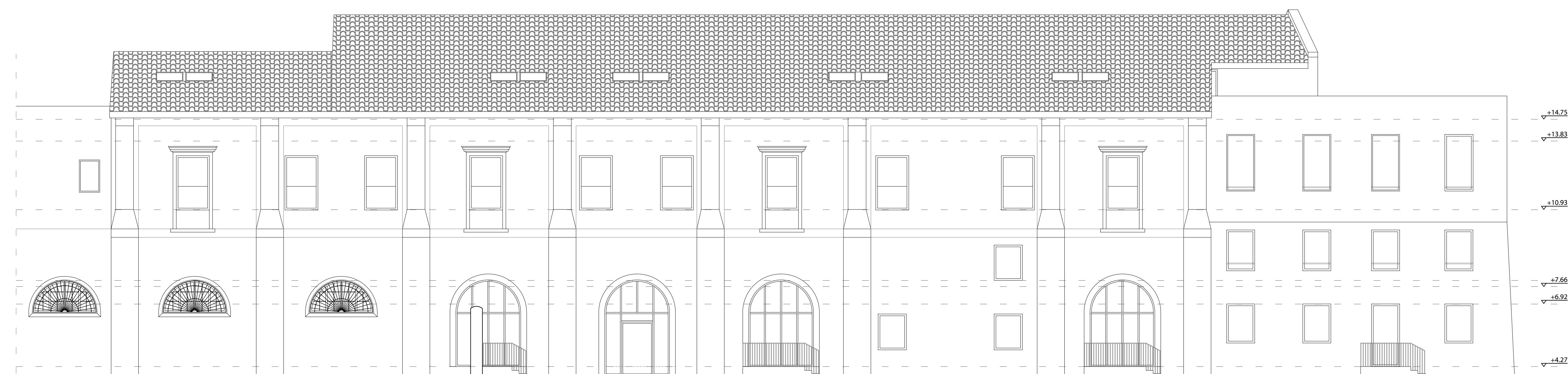
PROSPETTO NORD
