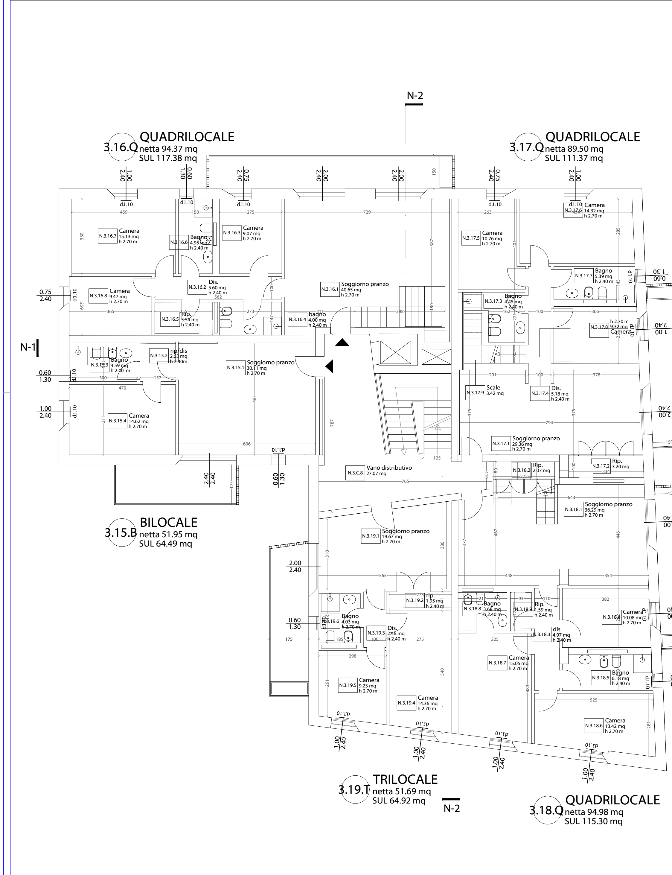
Stato di Progetto - ED_N - Piano Quarto
