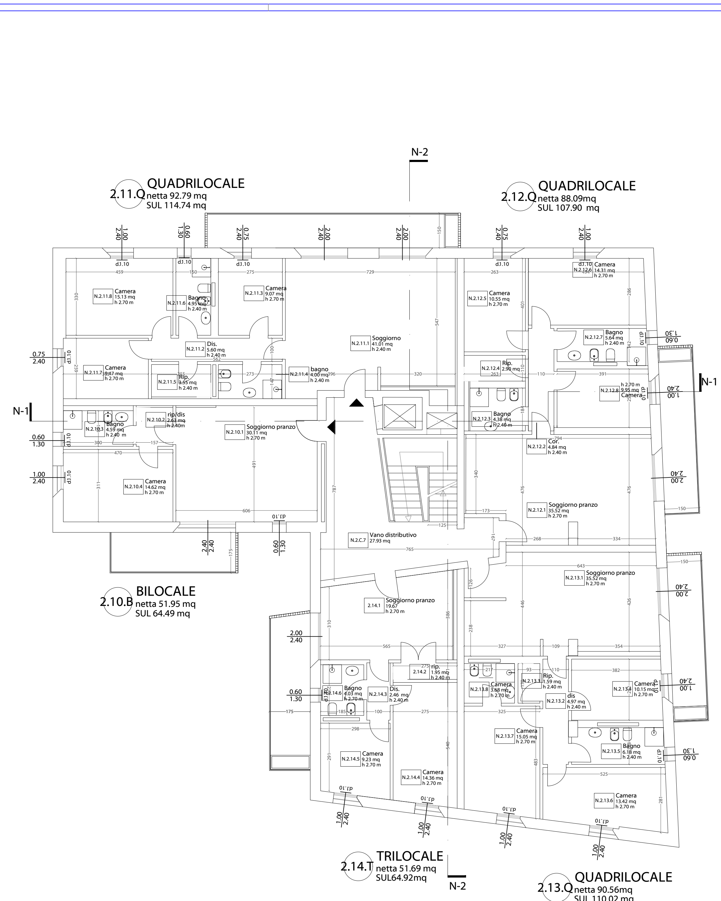
Stato di Progetto - ED_N - Piano Secondo
