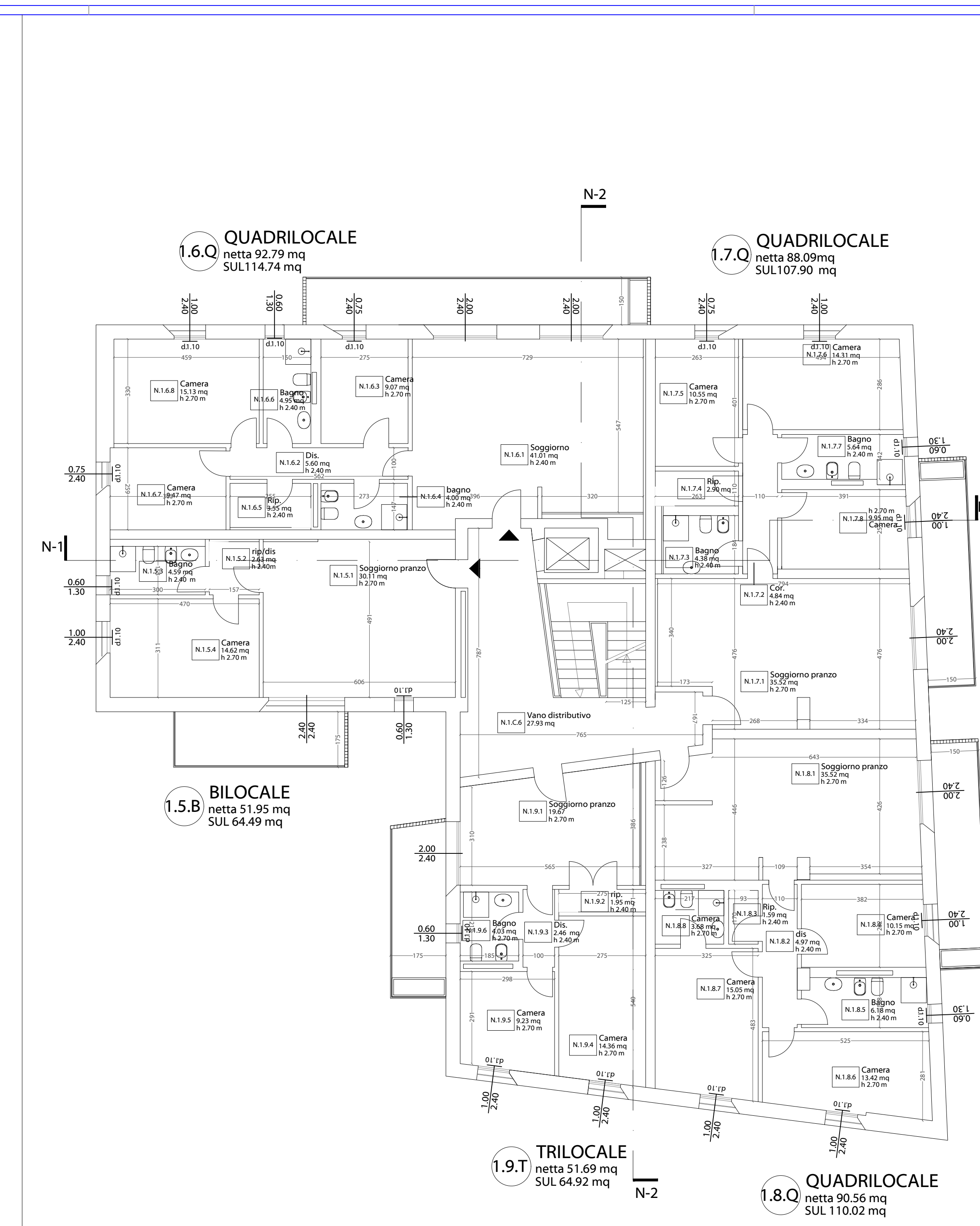
Stato di Progetto - ED_N - Piano Primo
