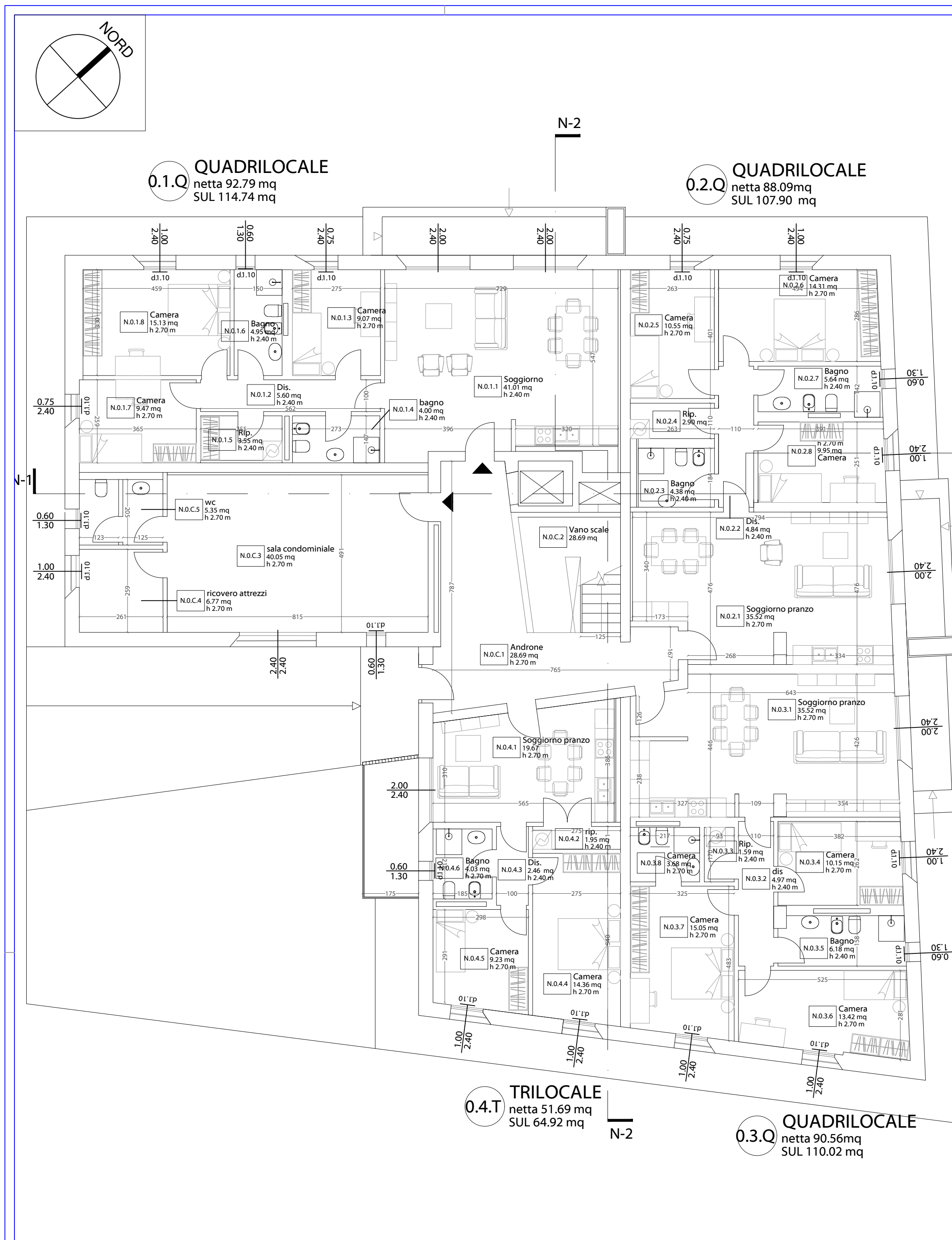
Stato di Progetto - ED_N - Piano Terra
