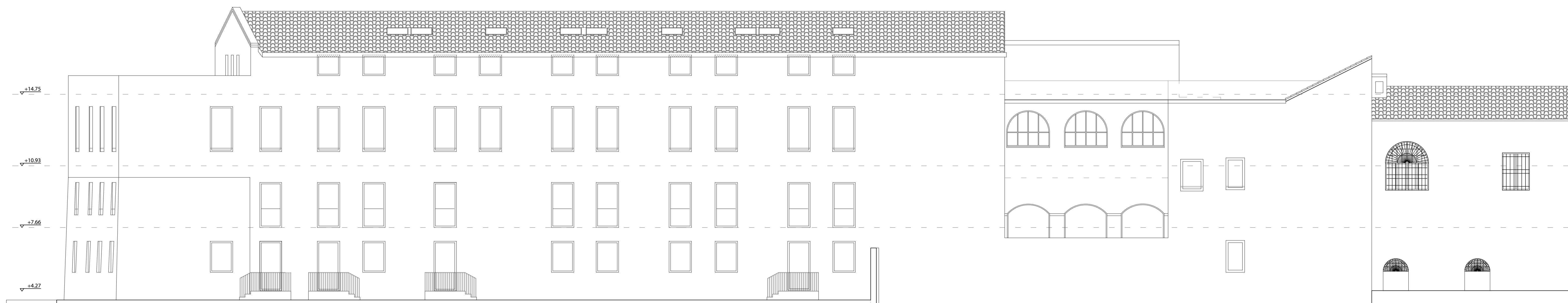
PROSPETTO SUD
