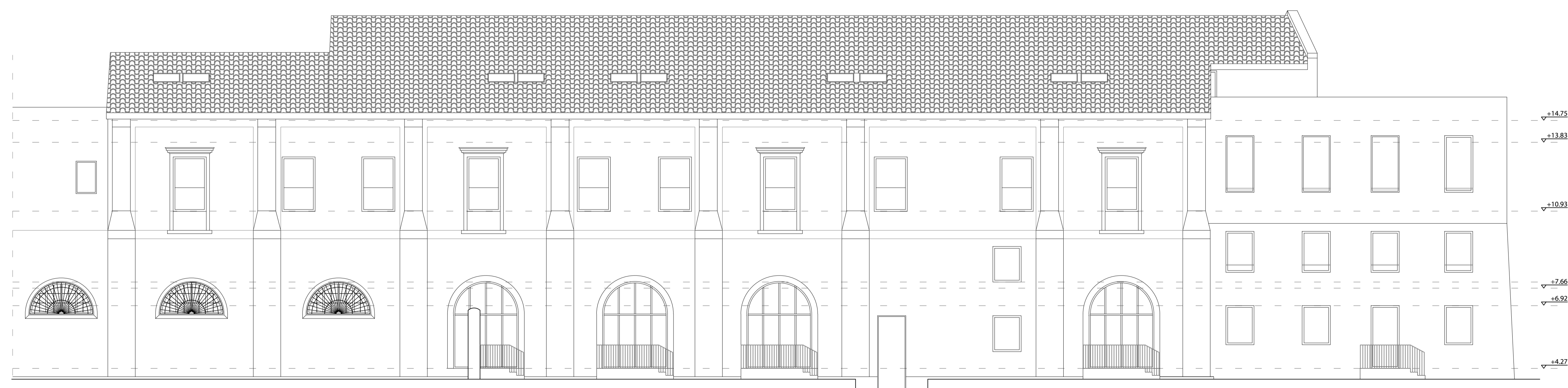
PROSPETTO NORD
