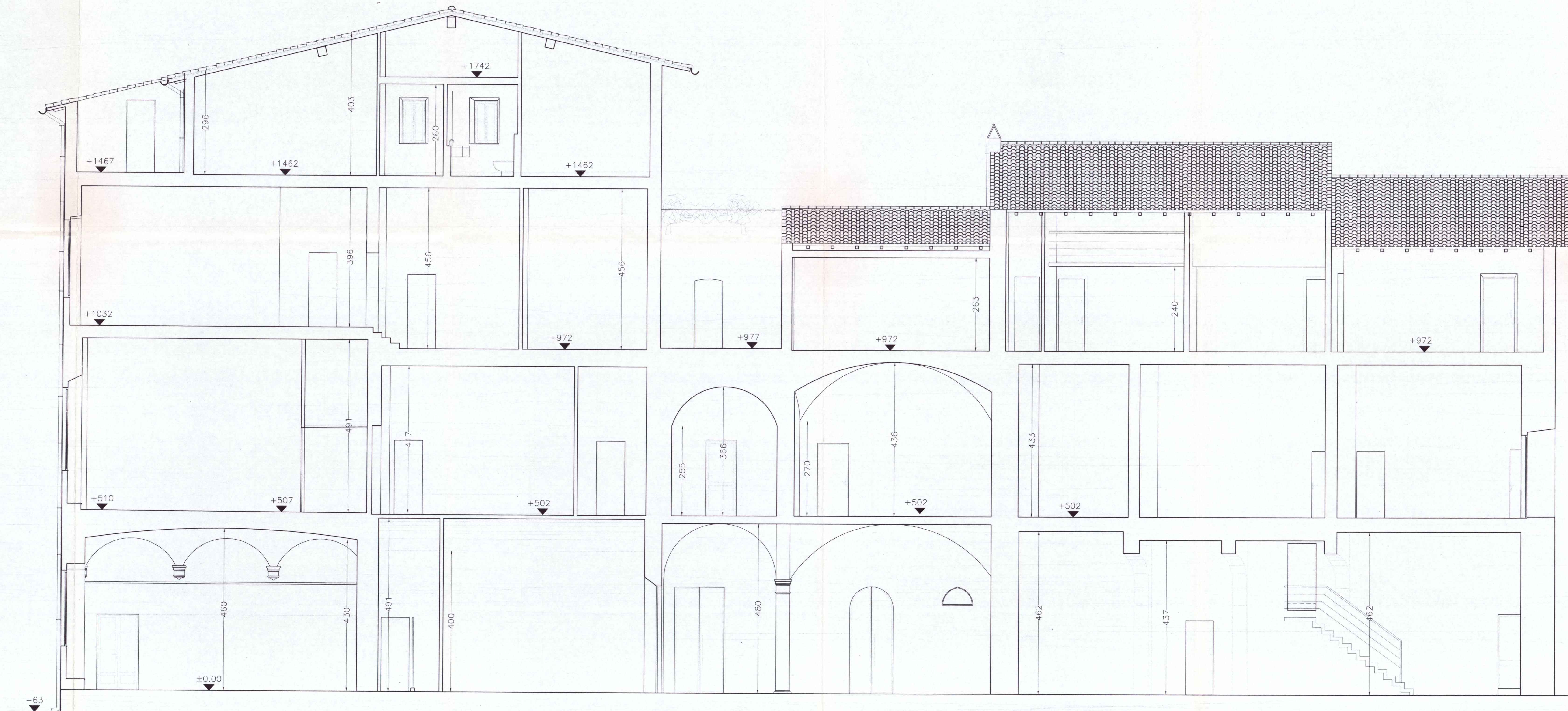
SEZIONE LONGITUDINALE A-A
