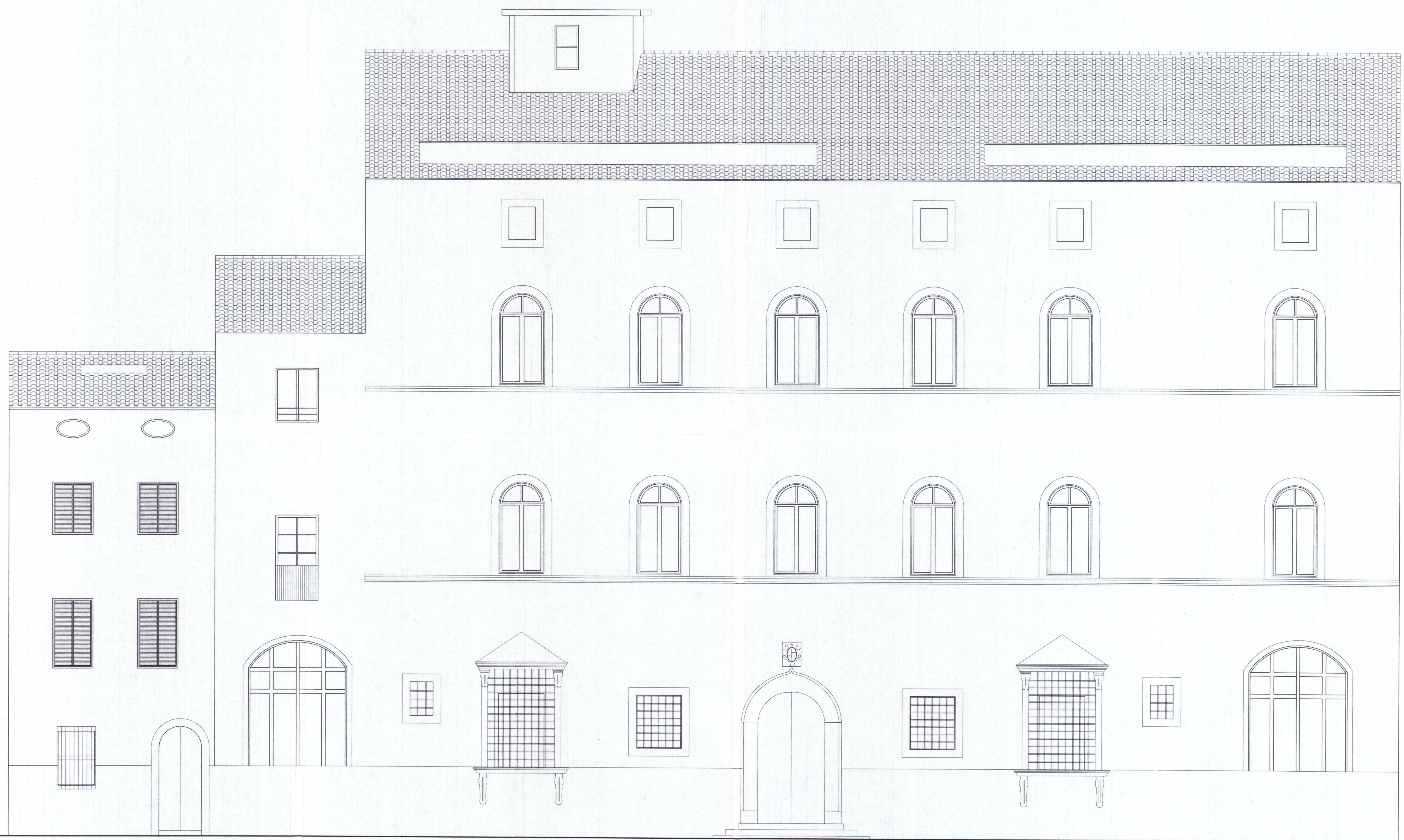
PROSPETTO OVEST VIA MAZZINI (A-A)
