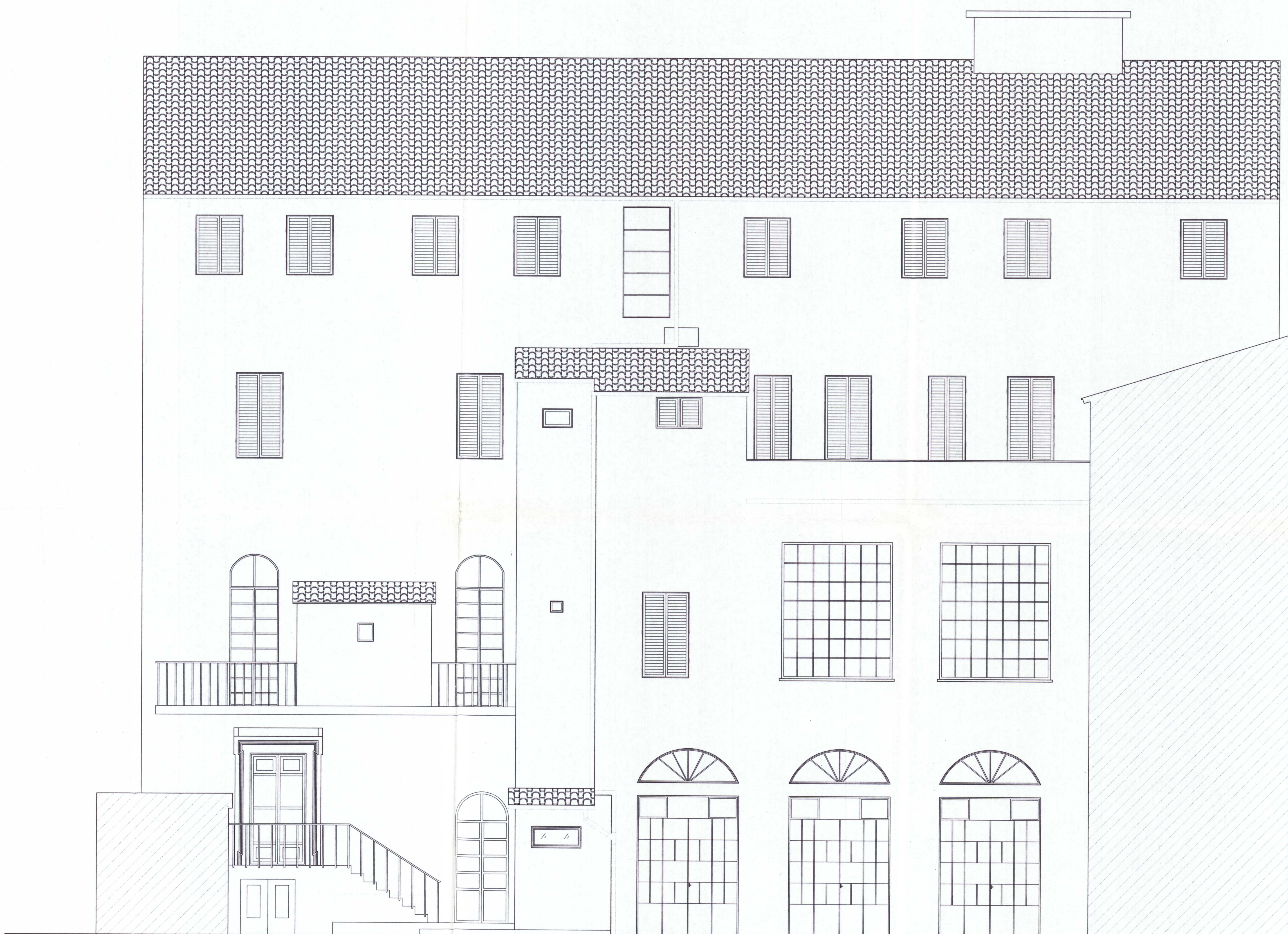
PROSPETTO EST CORTILE
