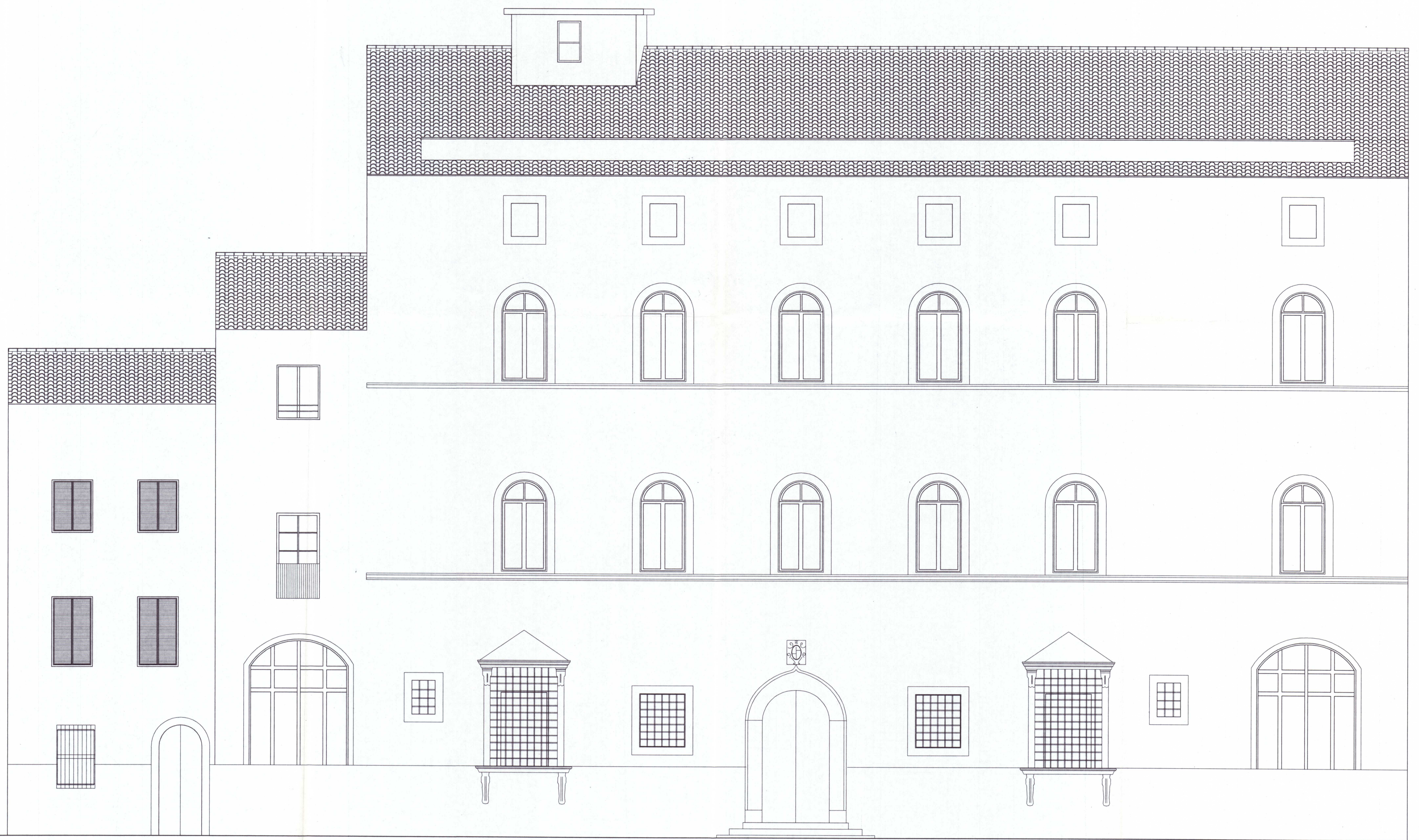
PROSPETTO OVEST VIA MAZZINI
