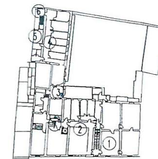
PIANTA SECONDO LIVELLO
