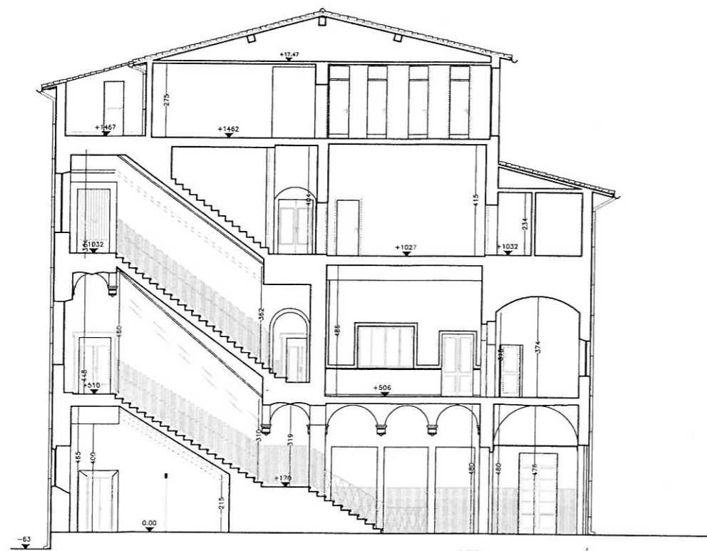
SEZIONE SCALE B-B
