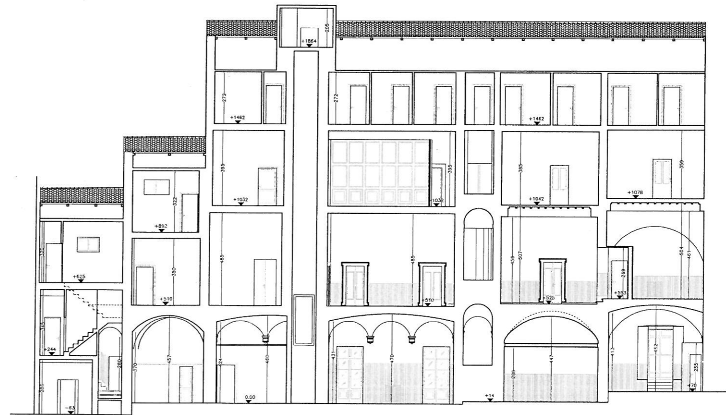
SEZIONE TRASVERSALE C-C
