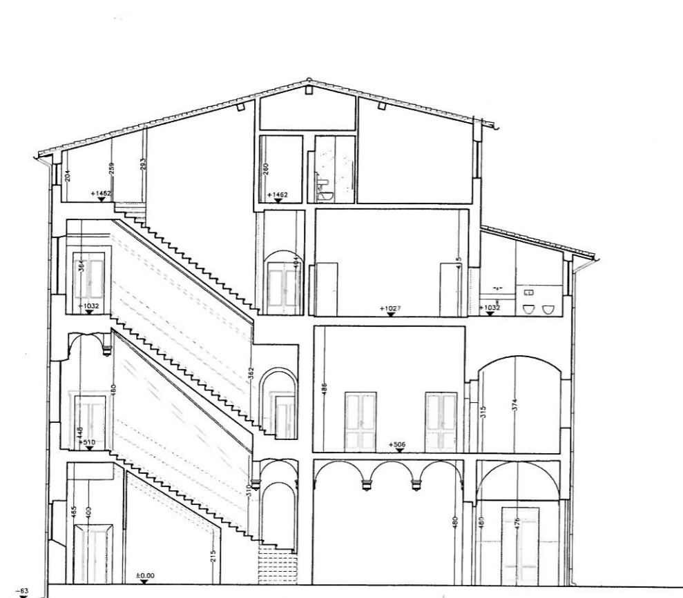
SEZIONE SCALE B-B
