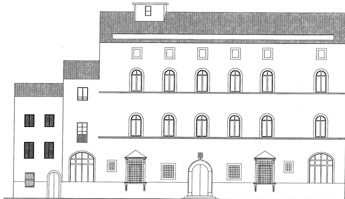
PROSPETTO OVEST VIA MAZZINI
