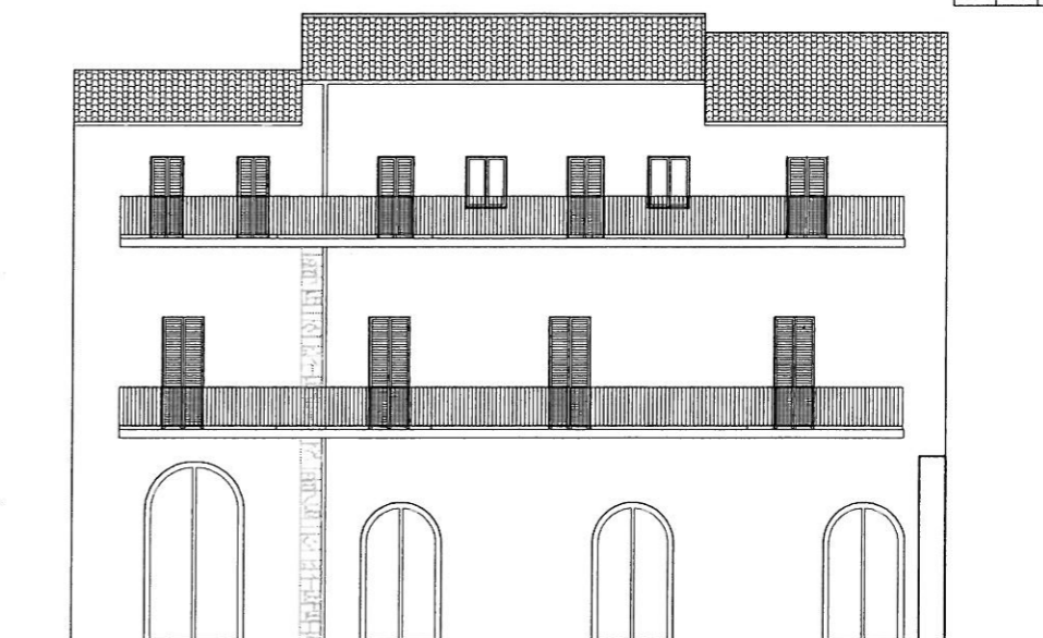
PROSPETTO NORD CORTILE
