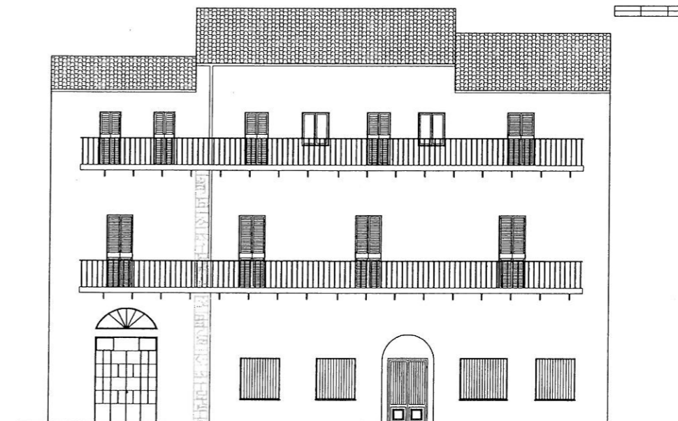
PROSPETTO NORD CORTILE A
