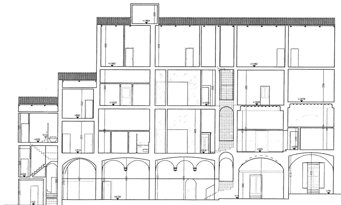
SEZIONE TRASVERSALE C-C
