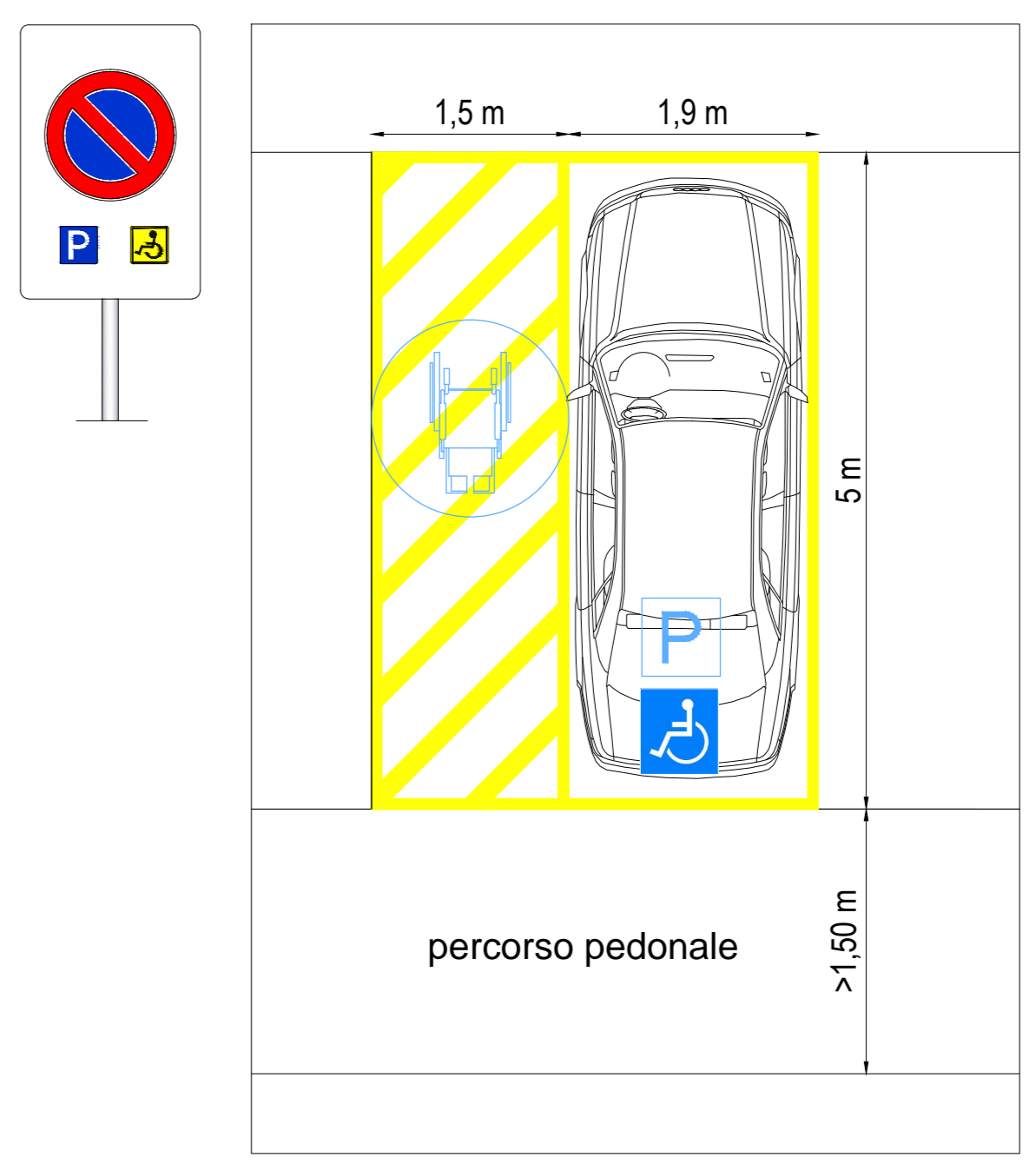
PARTICOLARE POSTO AUTO TIPO PER DISABILI
