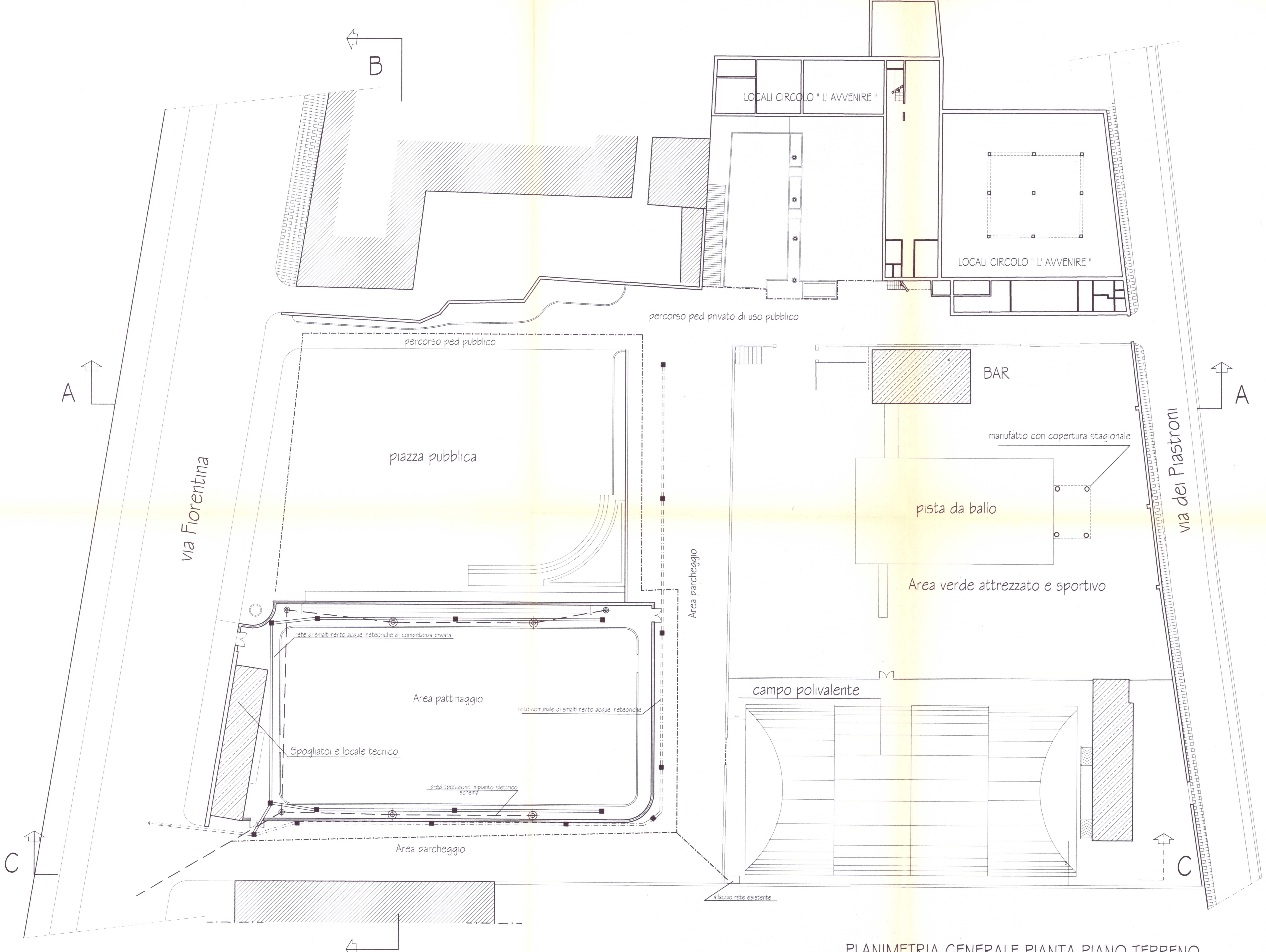
PLANIMETRIA GENERALE PIANTA PIANO TERRENO
