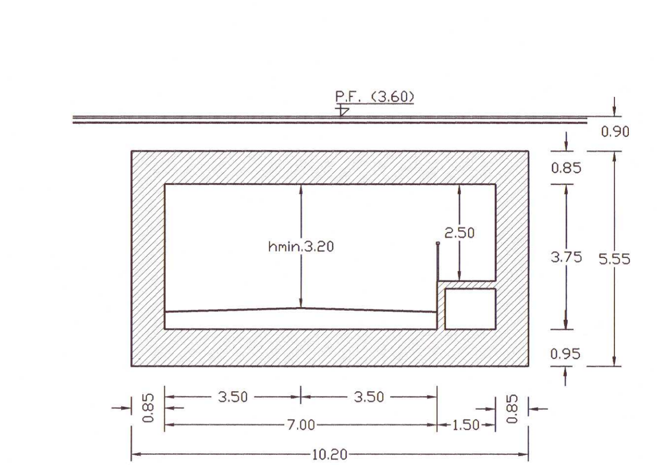
SEZIONE TRASVERSALE SOTTOVIA Scala 1:100
