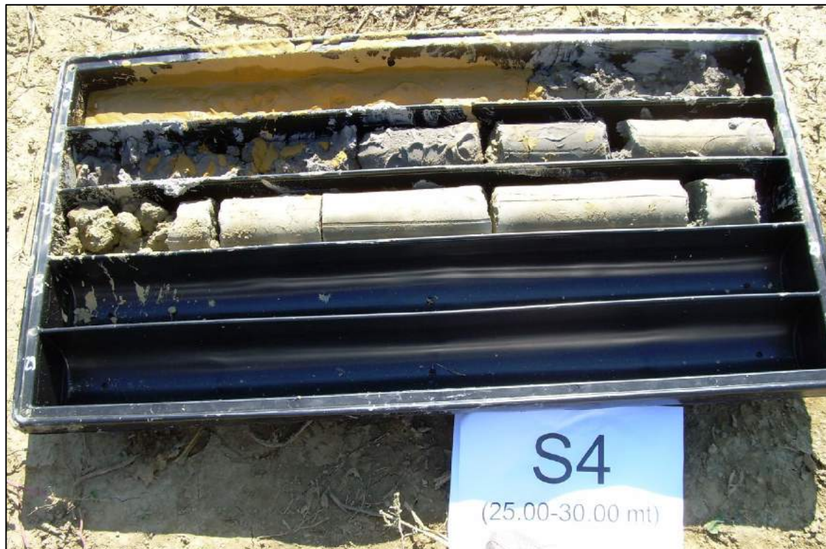
Sondaggio S4 (25.00-28.00)
