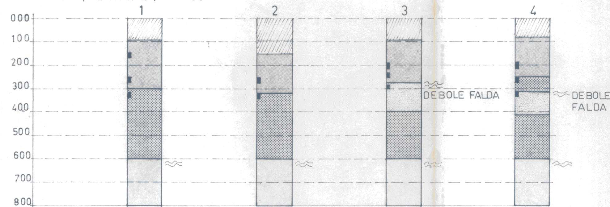
STRATIGRAFIE SCALA (VERTICALI) 1:100
