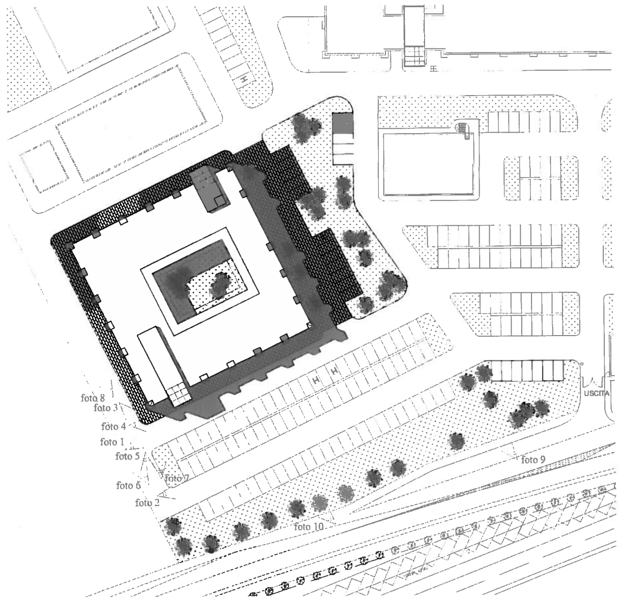
Planimetria generale con punti fotografici
