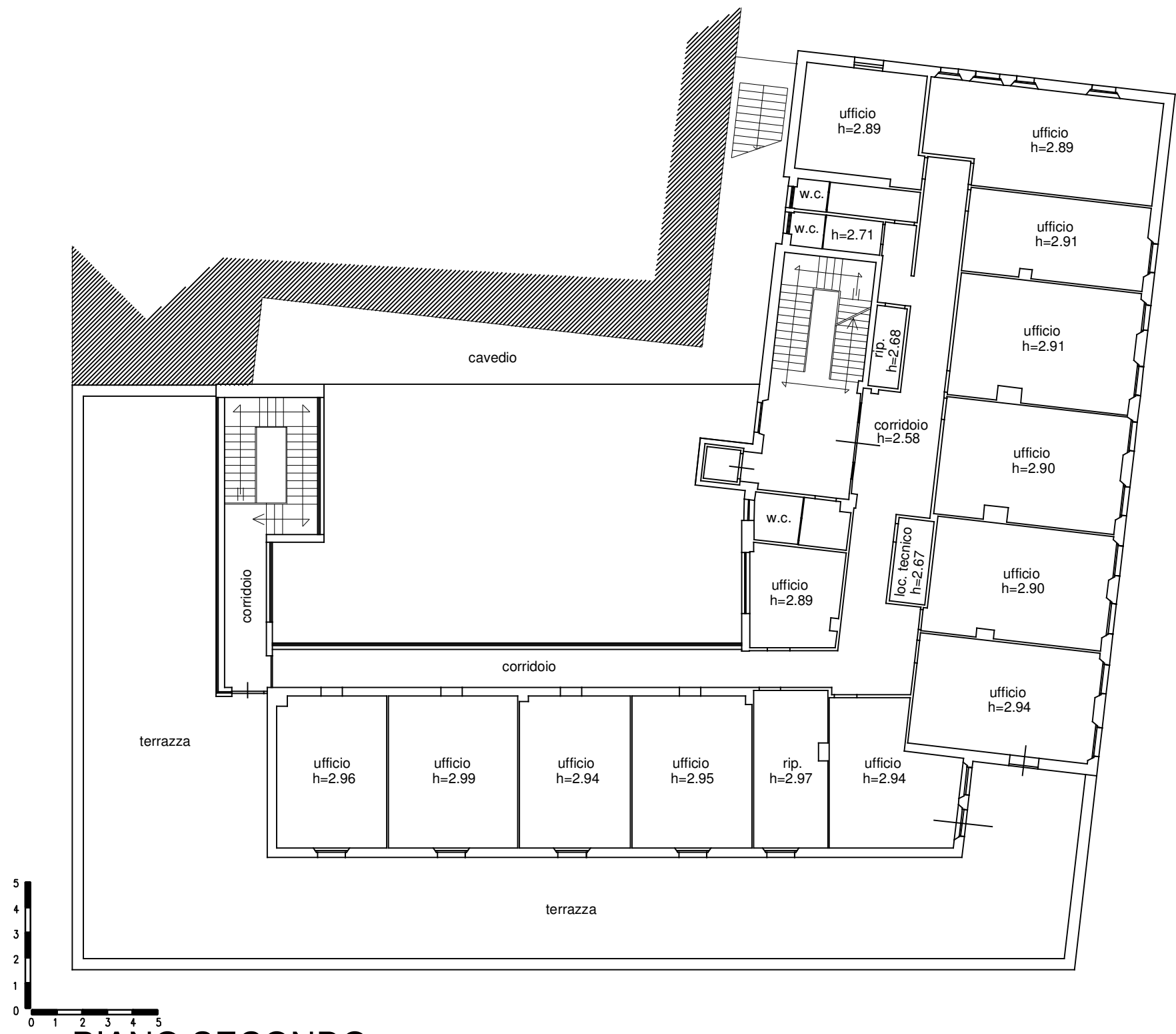
PIANO SECONDO
