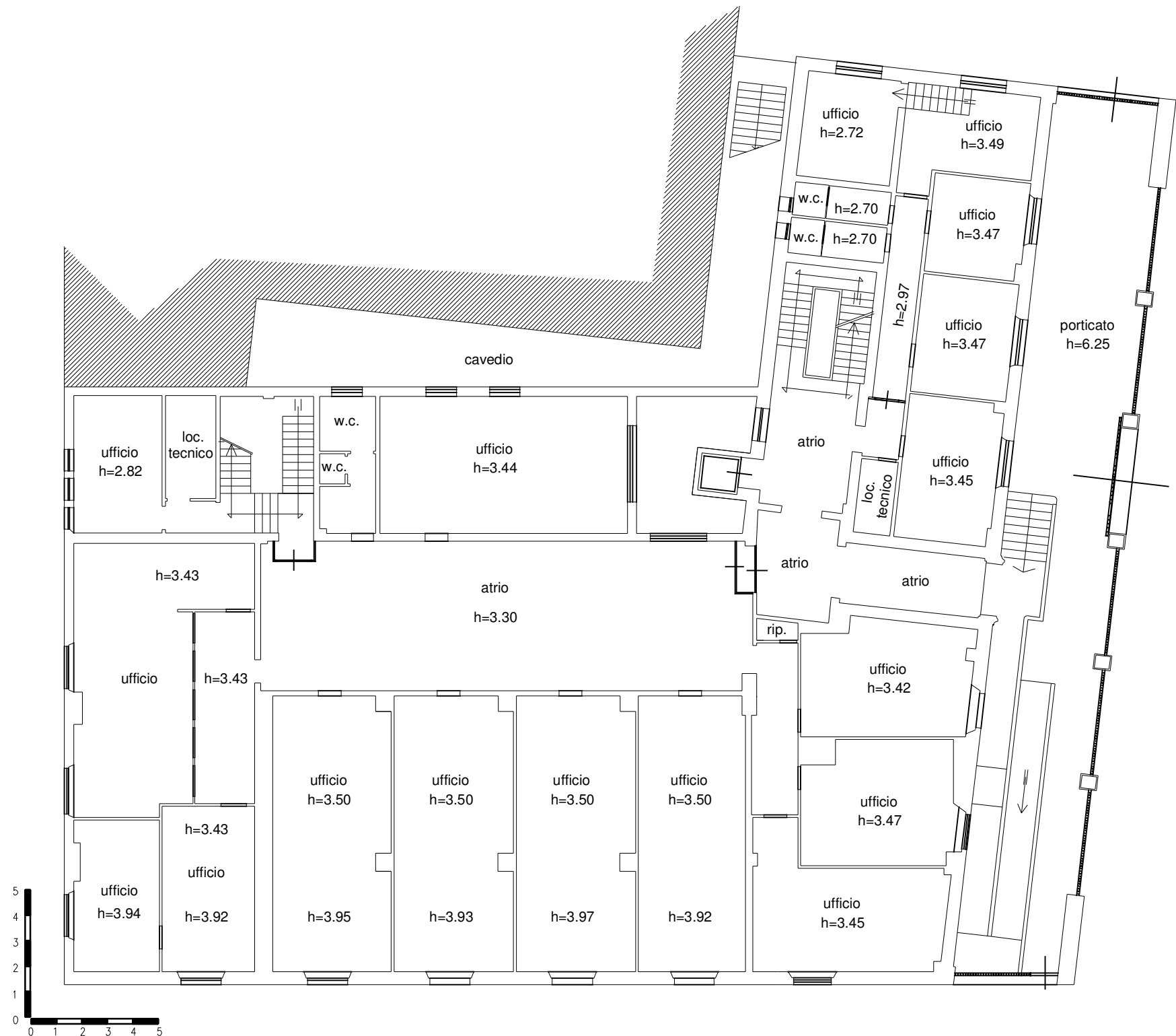
PIANO TERRA (RIALZATO)
