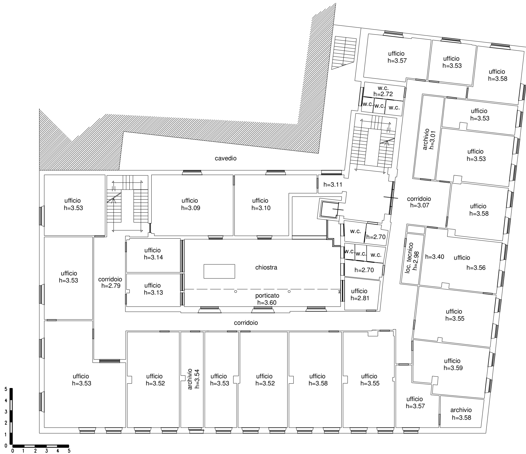
PIANO PRIMO
