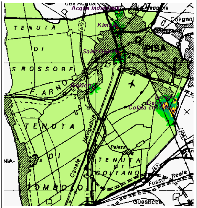
Lnight
