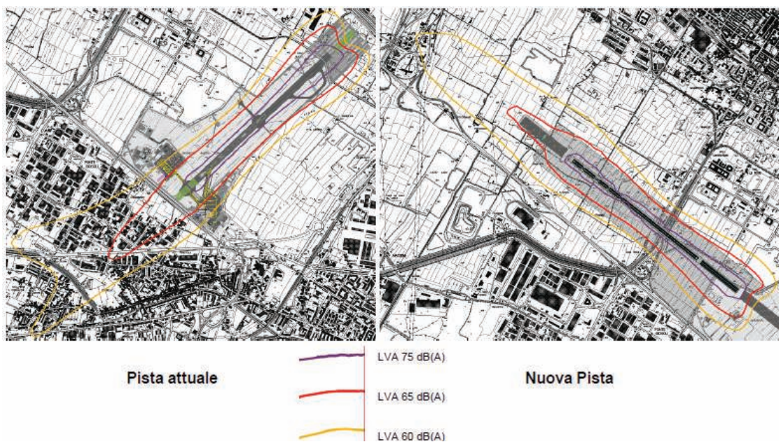
Figura 5.5 PROFILO DELLE CURVE ISOFONICHE NELLE DUE IPOTESI
