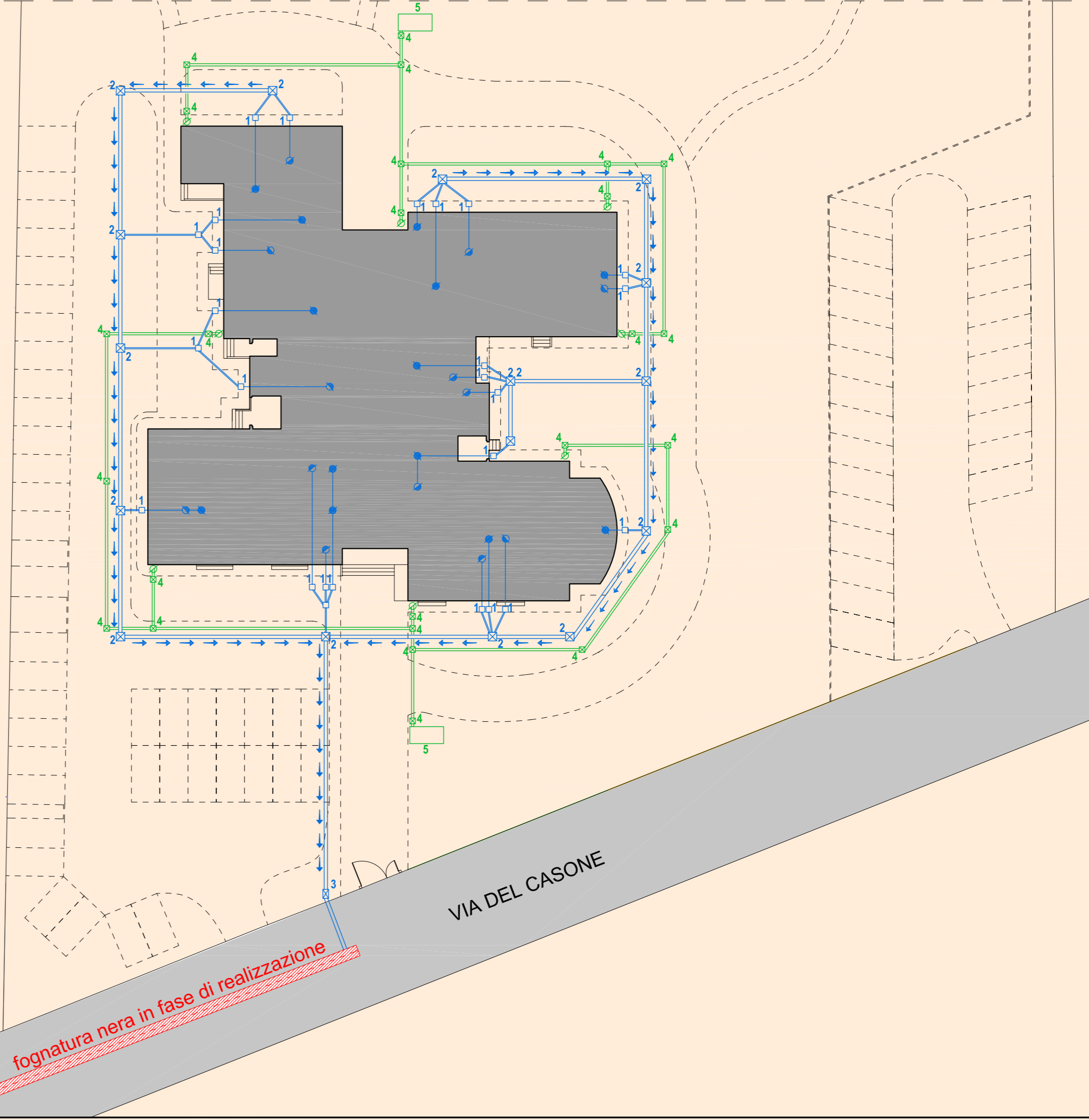
PLANIMETRIA STATO PROGETTO scala 1:200
