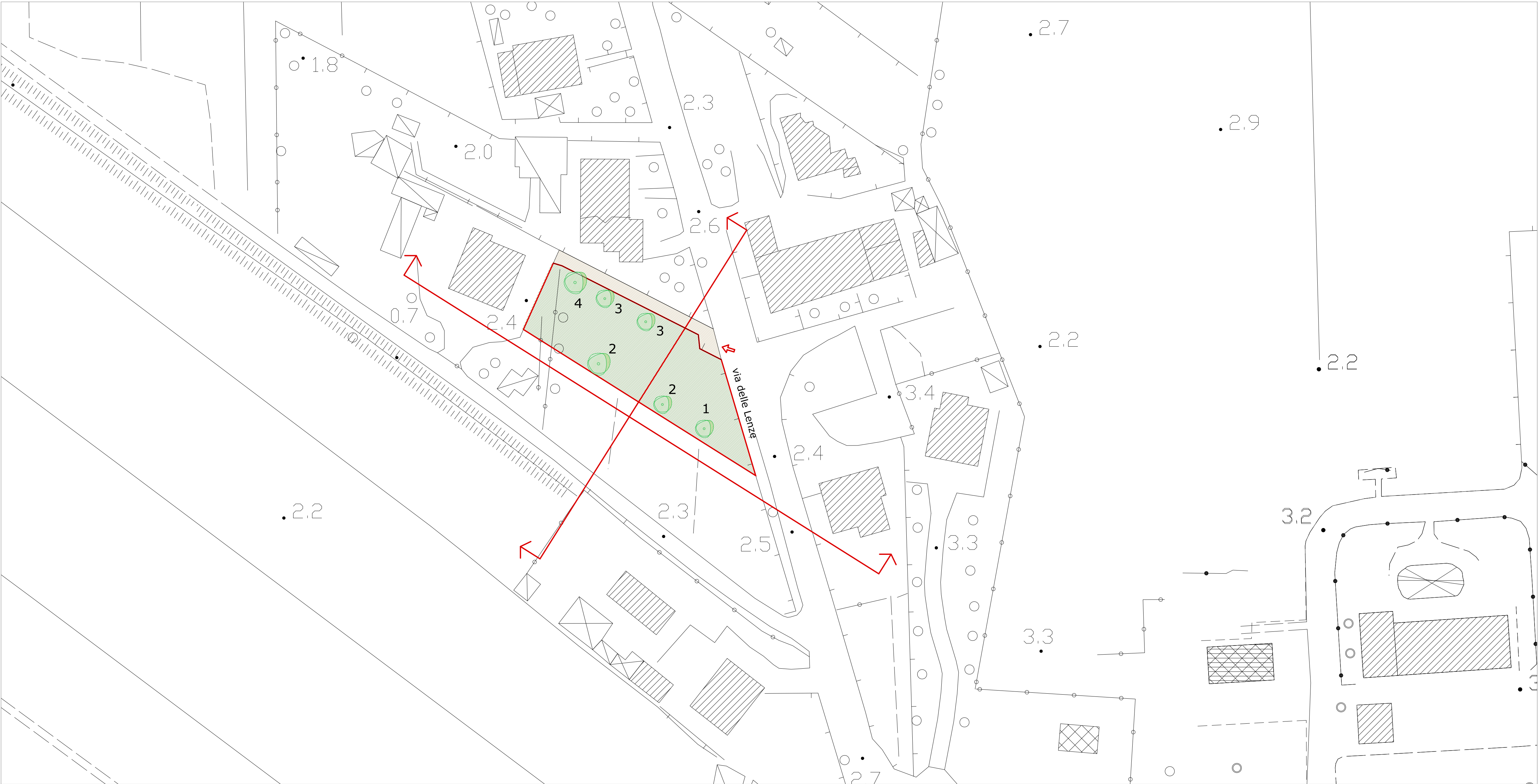
PLANIMETRIA GENERALE CTR
