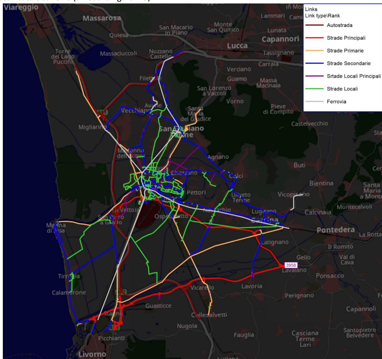
Figura 4.5 – La rete di trasporto multimodale
