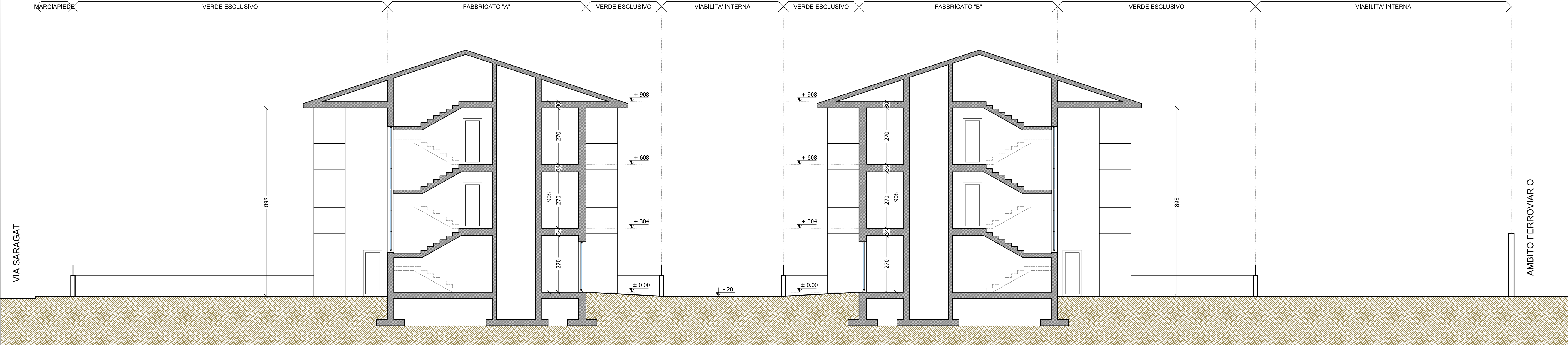
SEZIONE A-A
