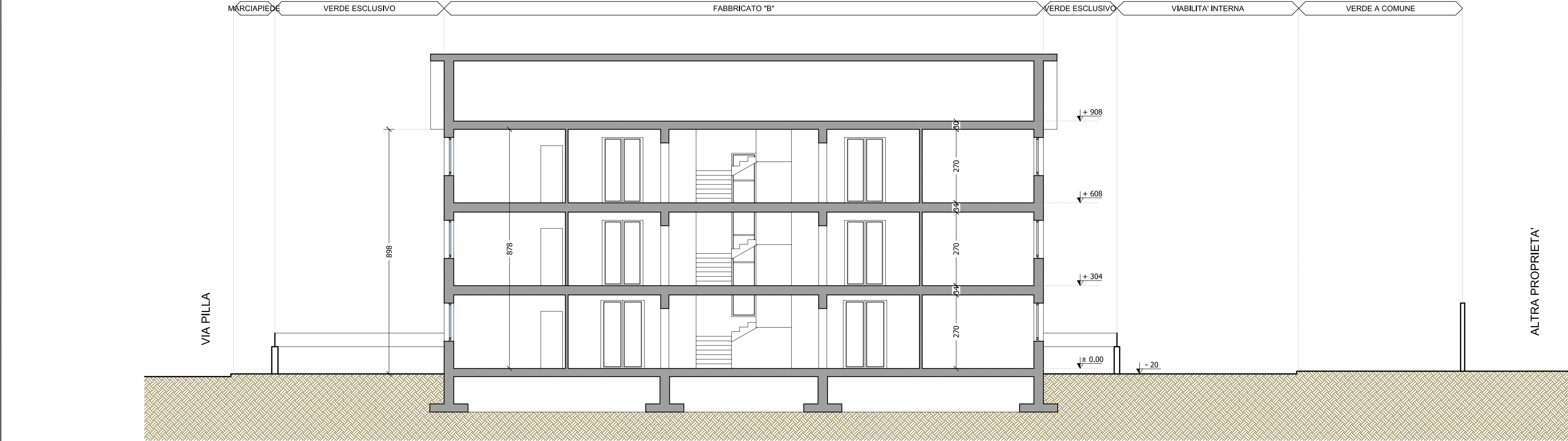
SEZIONE B-B
