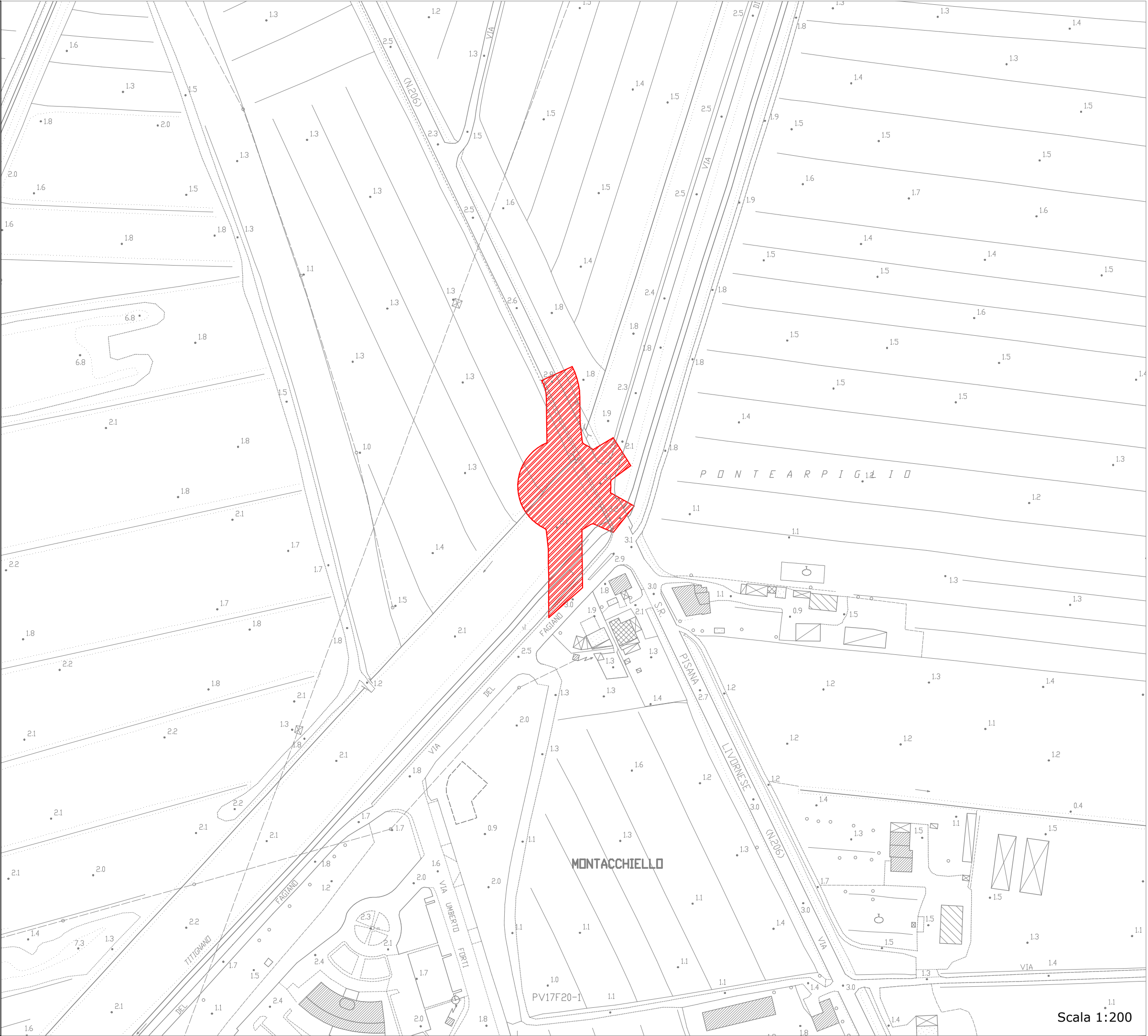
Tavola 10: Progetto per la realizzazione di rotatoria all'intersezione tra Via Emilia, Via del Fagiano e Via di Titignano nel Comune di Cascina.
