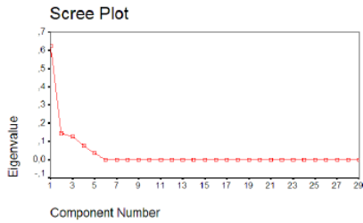
Fig. 1.6. Screplot dell'estrazione degli auto valori associati a ciascun fattore estratto.
