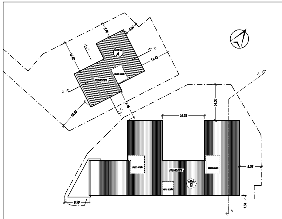
Plani 1° e 2° - Edifici A e B
