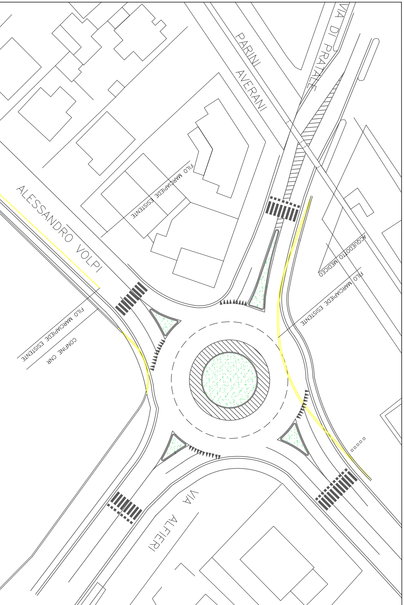
Fig. 2.8 -Rotatoria nel nodo via Di Pratatale - via Volpi-Via Alfieri
