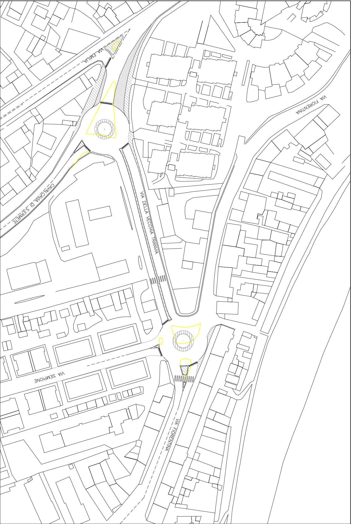
Fig.2.4 - Progetto di due minirotatorie in via della Vecchia Tranvia
