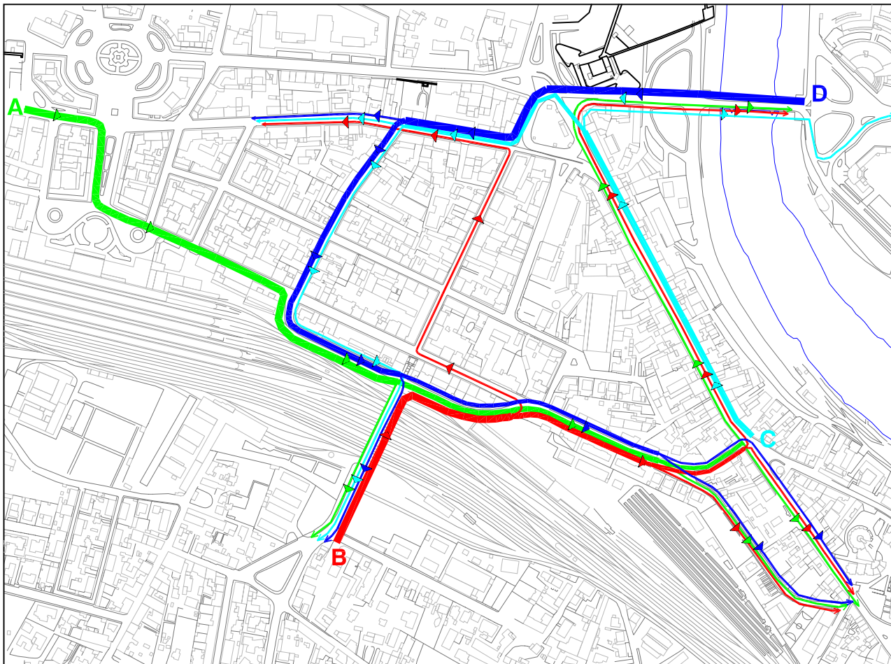
Fig. 2.2 a - scenario attuale
