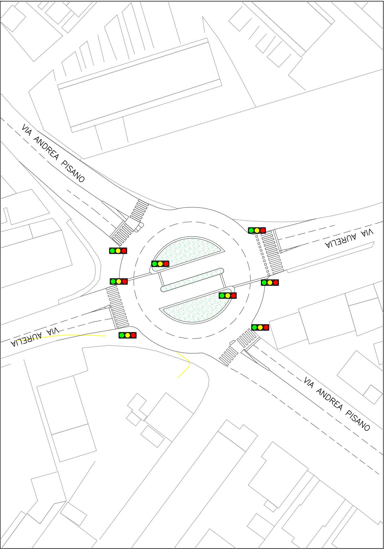
Fig. 2.16 - Rotatoria semaforizzata via Aurelia - via Andrea Pisano
