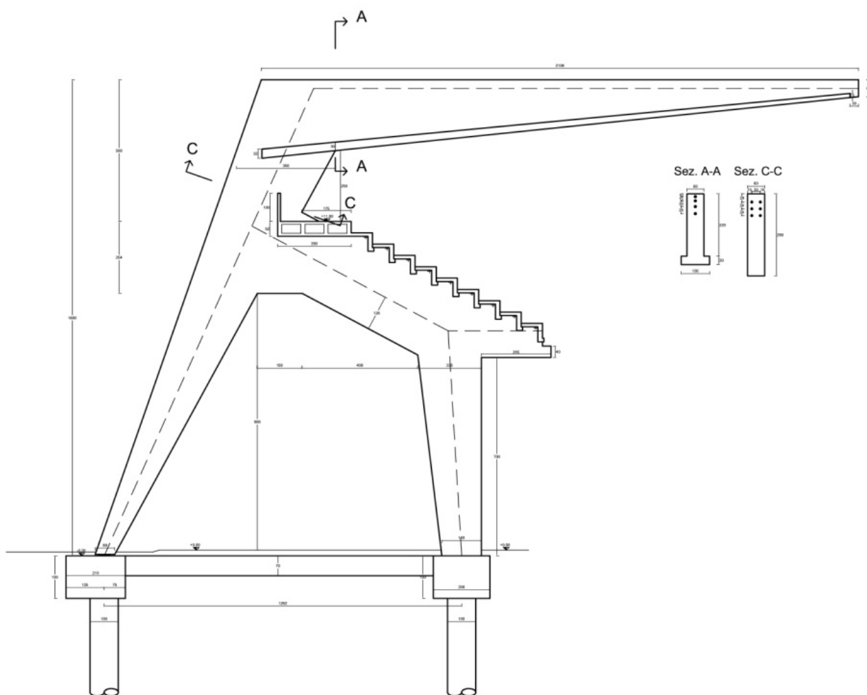
Figura 6.49 – Sezione Portale Tipo
