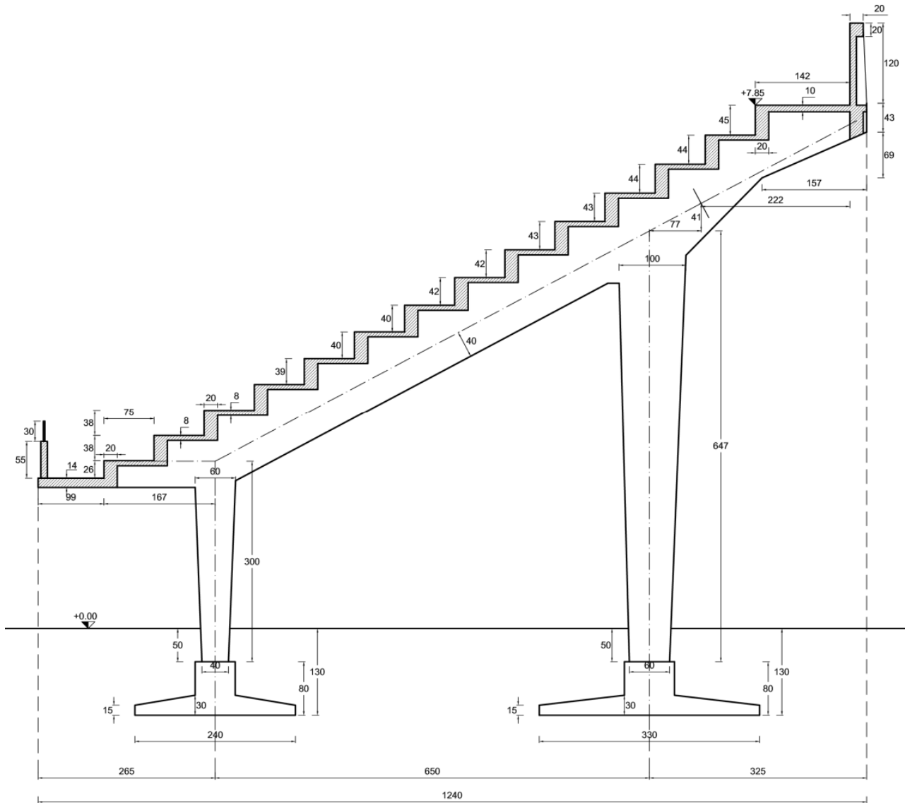
Figura 6. 18– Portale Tipo Curva Nord
