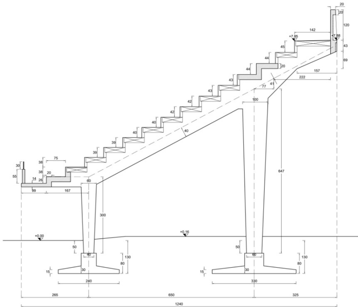
Figura 6.25 – Sezione Tipo Portali Gradinata – Curva Sud
