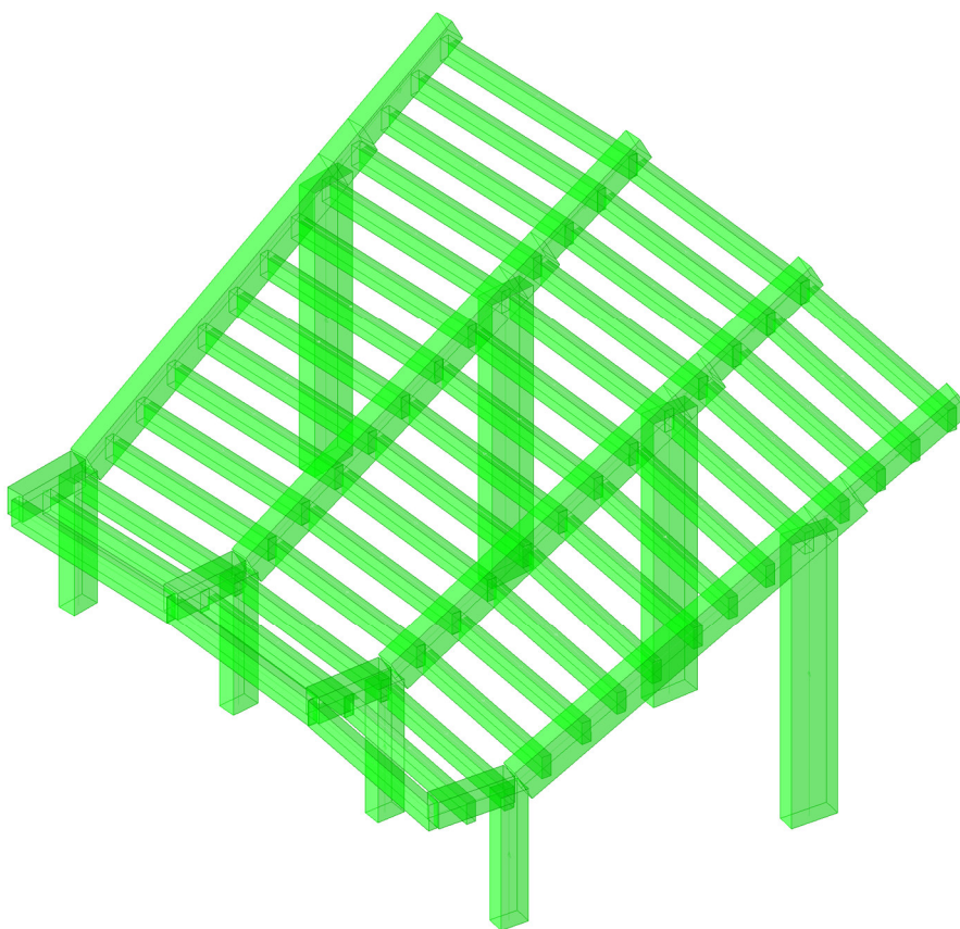
Figura 7.16 – Verifiche SLU per i soli carichi verticali (NTC2008)
