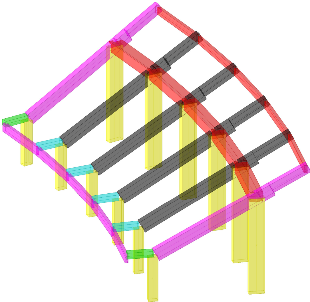
Figura 6.34 – Vista estrusa modello Corpo C-11
