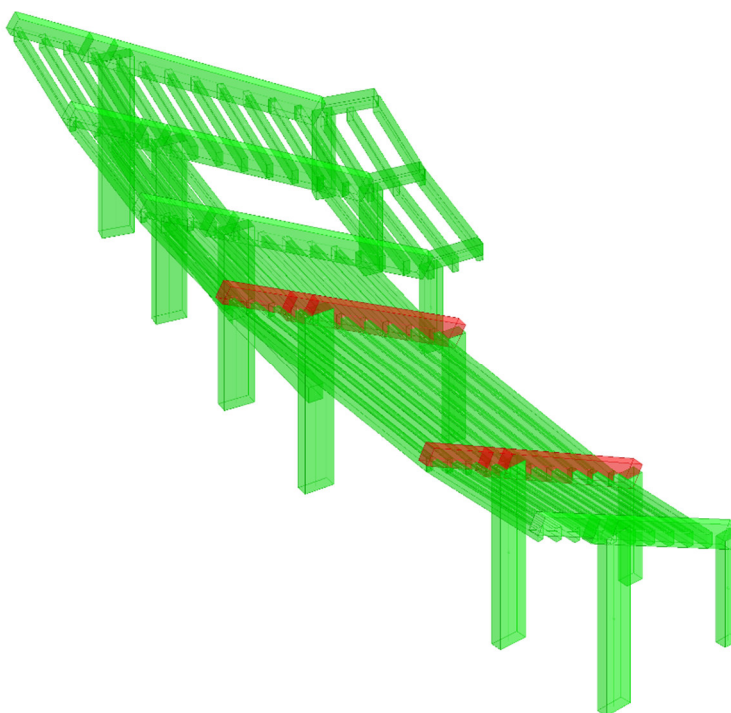
Figura 7.4 – Verifiche SLU per i soli carichi verticali (NTC2008)
