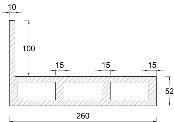
Figura 6.55 – Solaio camminamento superiore
