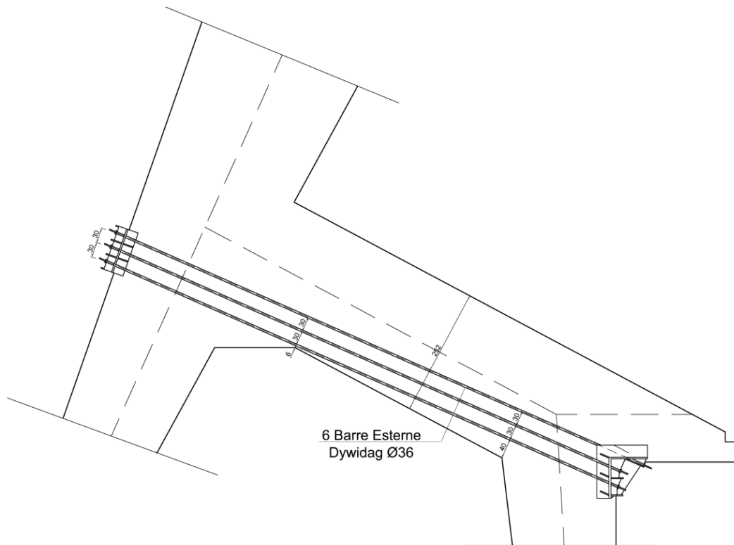
Figura 6.50 – Precompressione traversa
