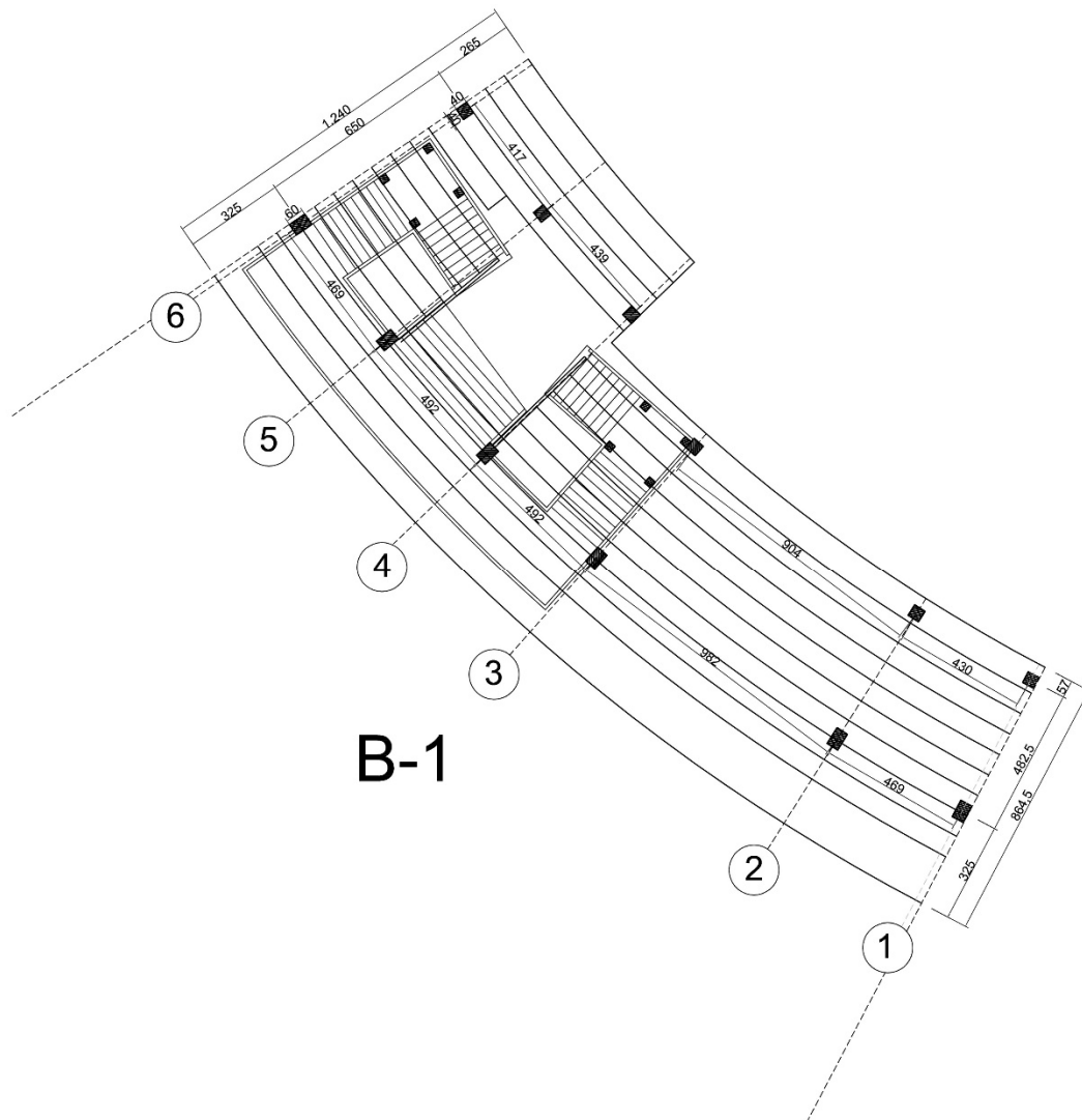
Figura 6.12 – Pianta Corpo B-1
