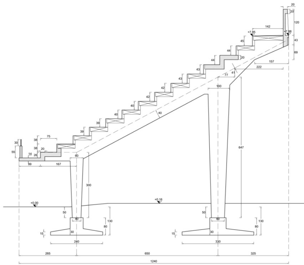
Figura 4.20 – Sezione tipo portale Gradinata – Curva Sud
