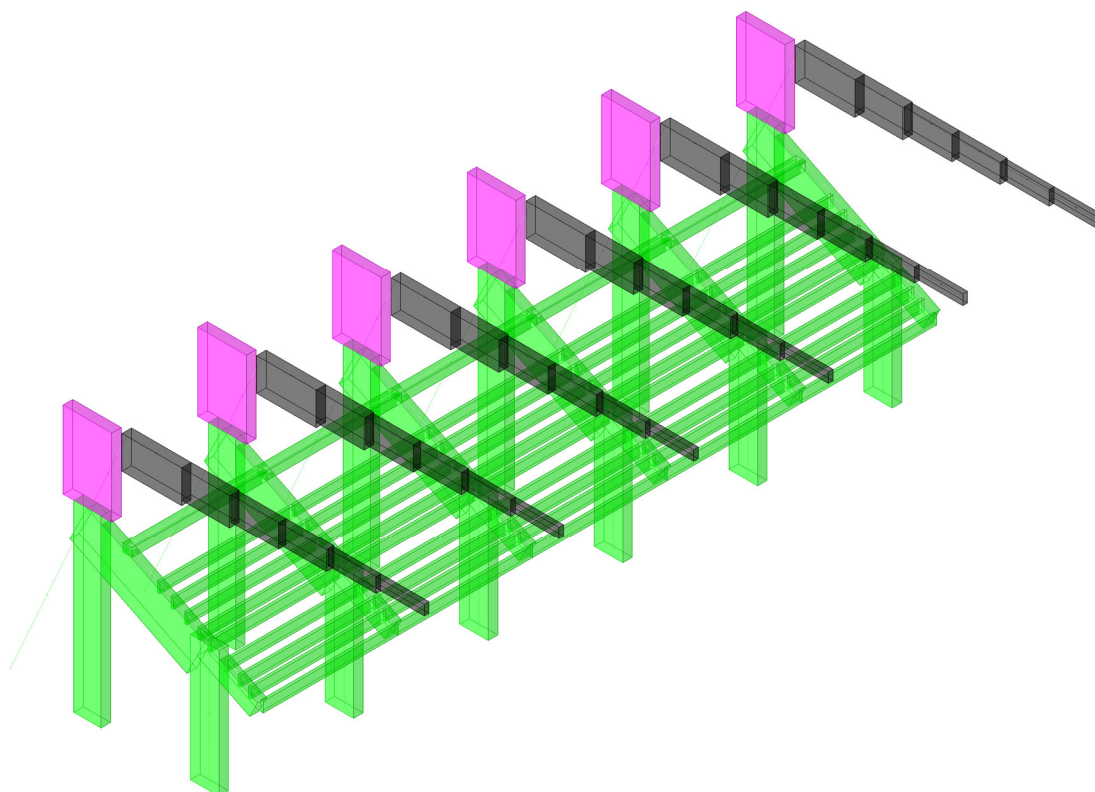
Figura 7.18 – Verifiche SLU per i soli carichi verticali (NTC2008)
