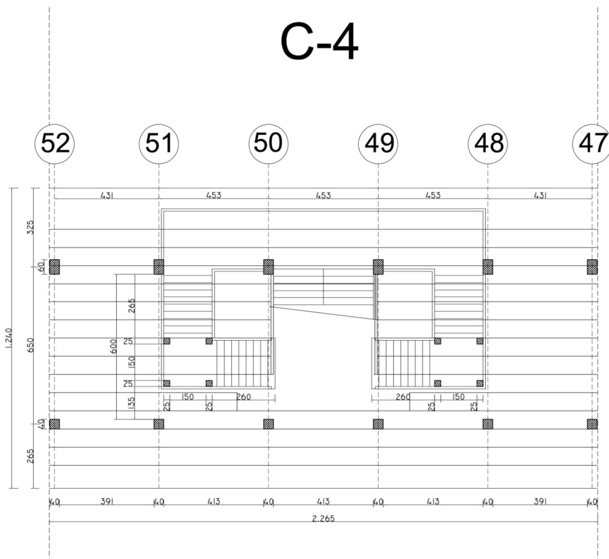
Figura 6.32 – Pianta Corpo C-4
