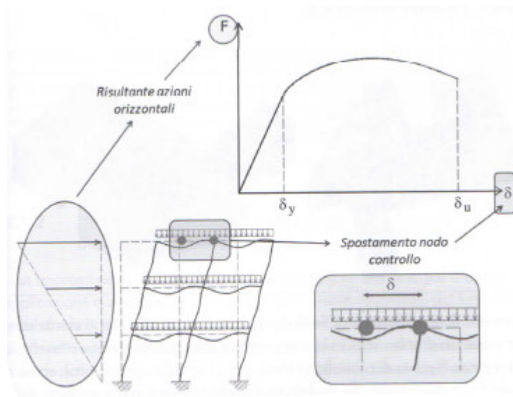
Figura 3.1 – Rappresentazione schematica curva di capacità
