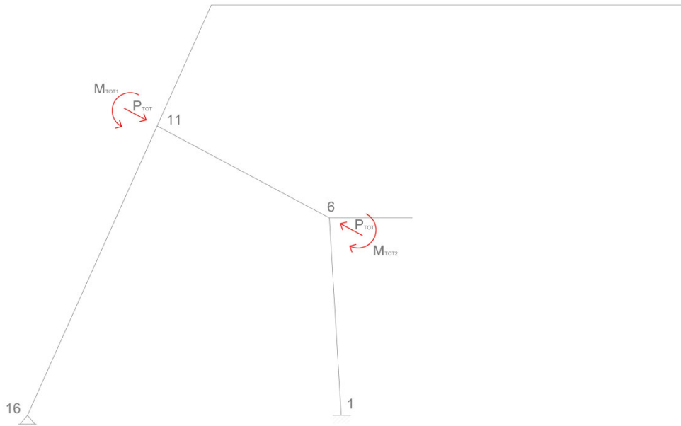
Figura 6.59 – Carichi Precompressione Esterna
