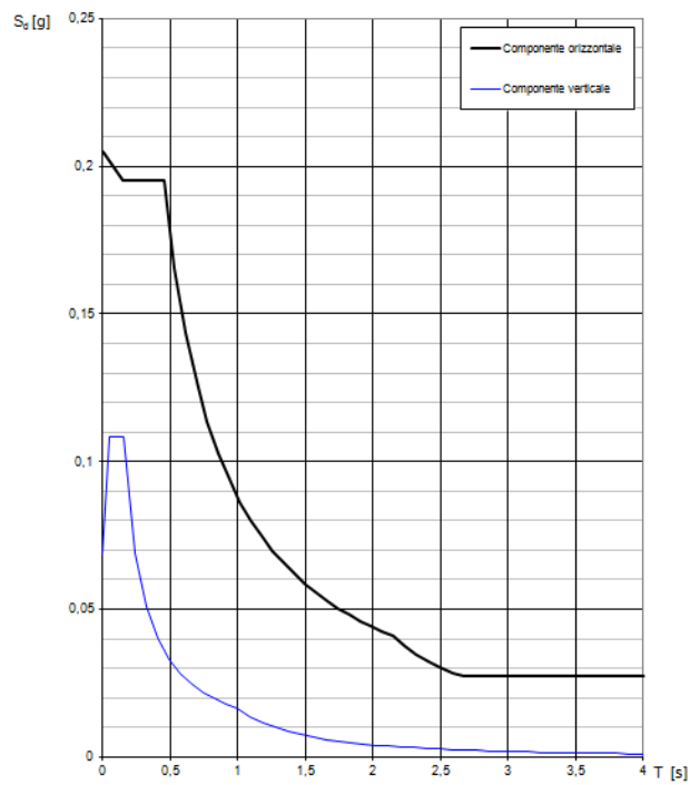
Figura 6.46 – Spettri SLV q = 2,5
