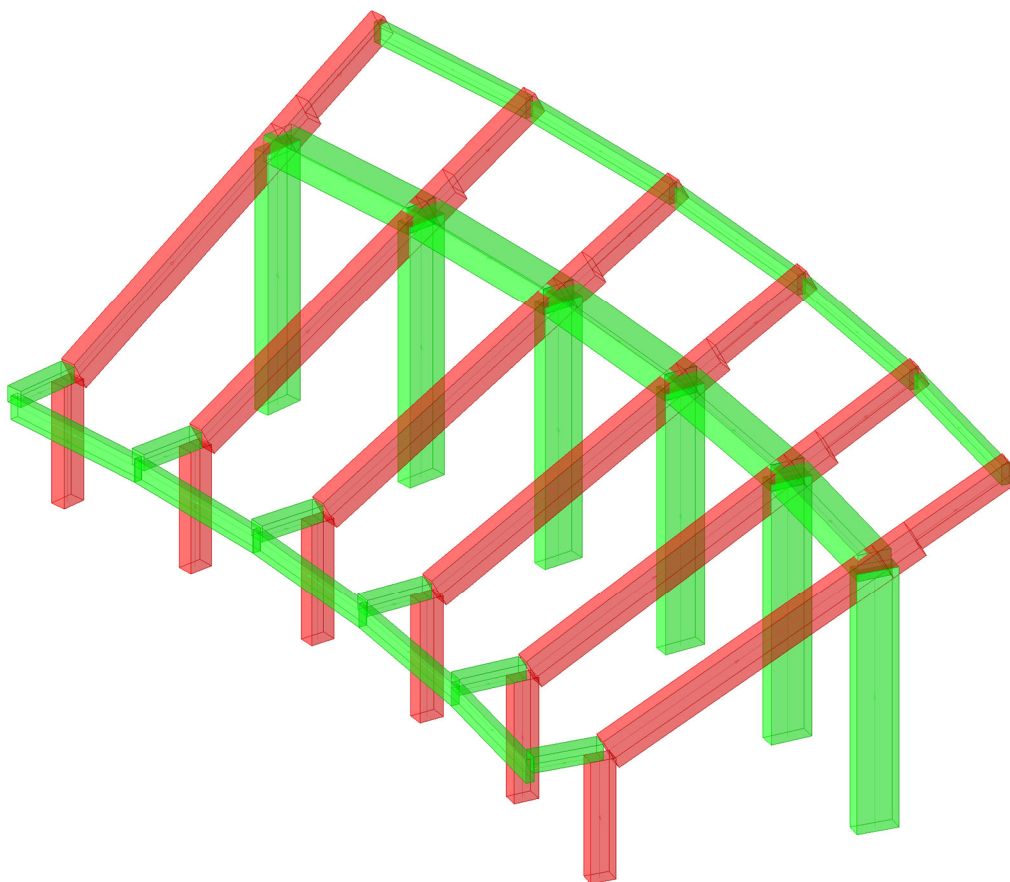
Figura 7.11 – Verifiche SLV Corpo C-11
