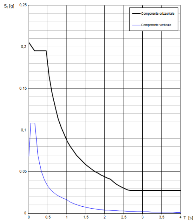
Figura 6.7 – Spettri SLV q = 2,5
