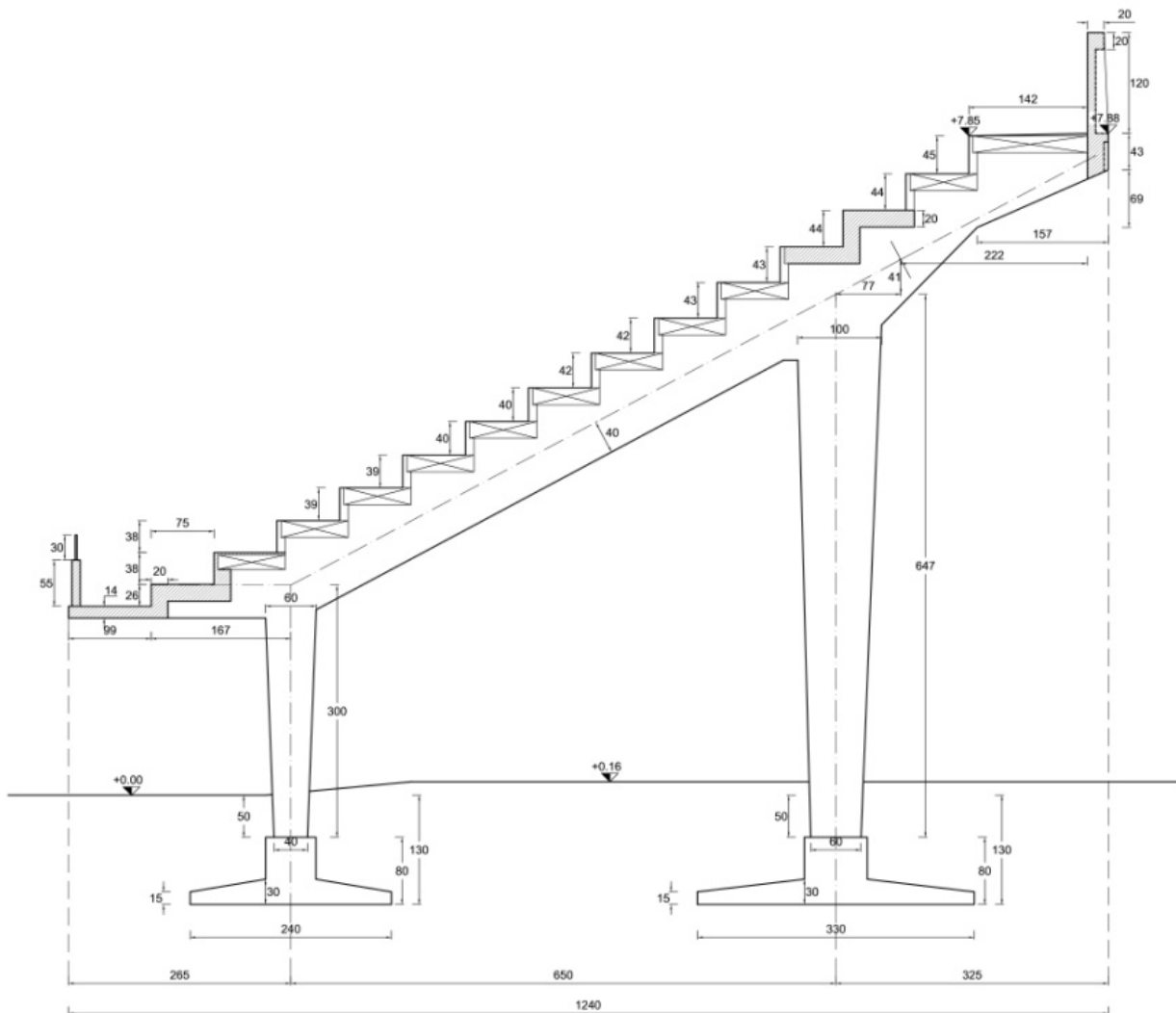
Figura 6.27 – Sezione Tipo Portali Gradinata – Curva Sud
