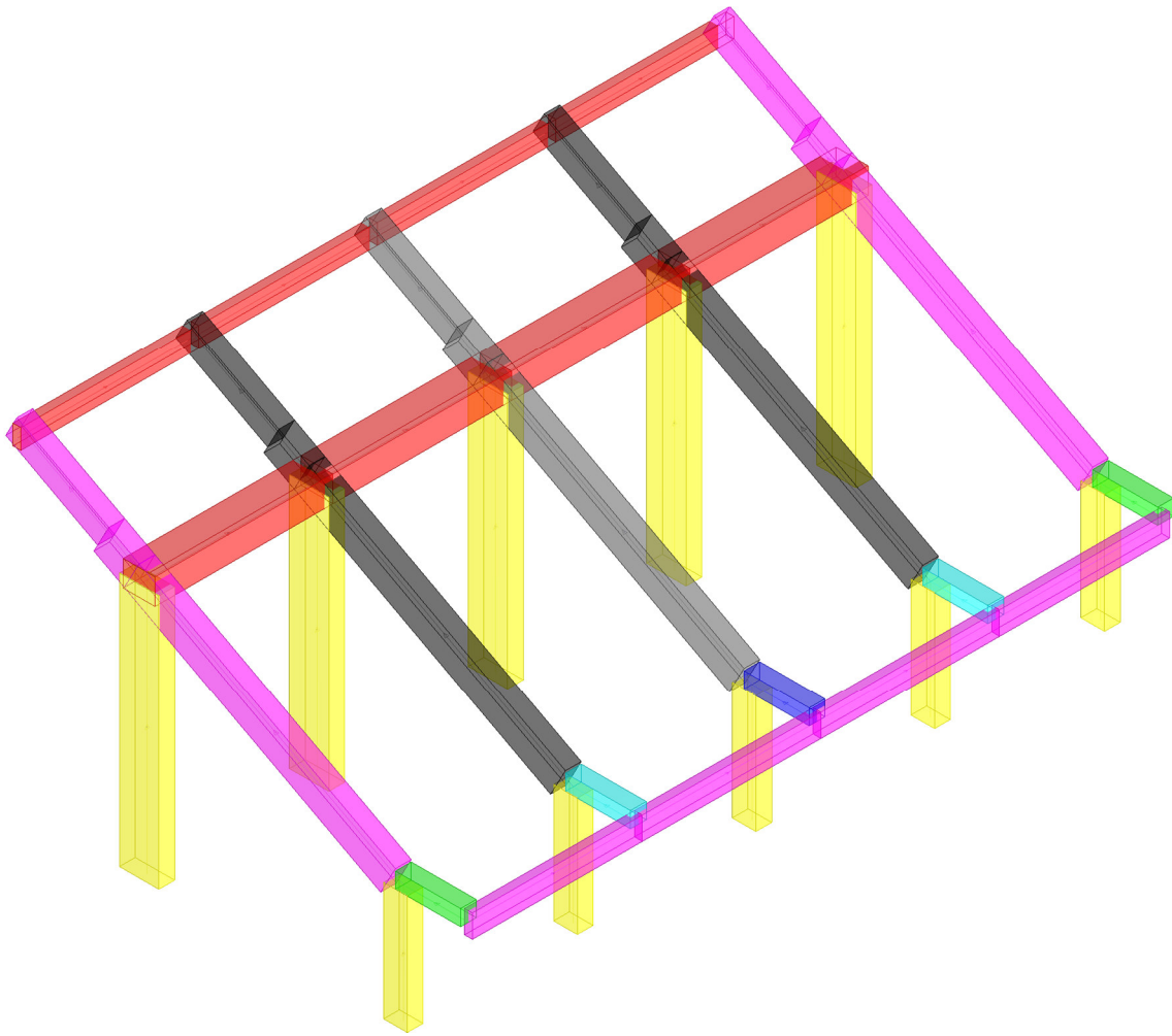
Figura 6.31– Vista estrusa modello Corpo C-3
