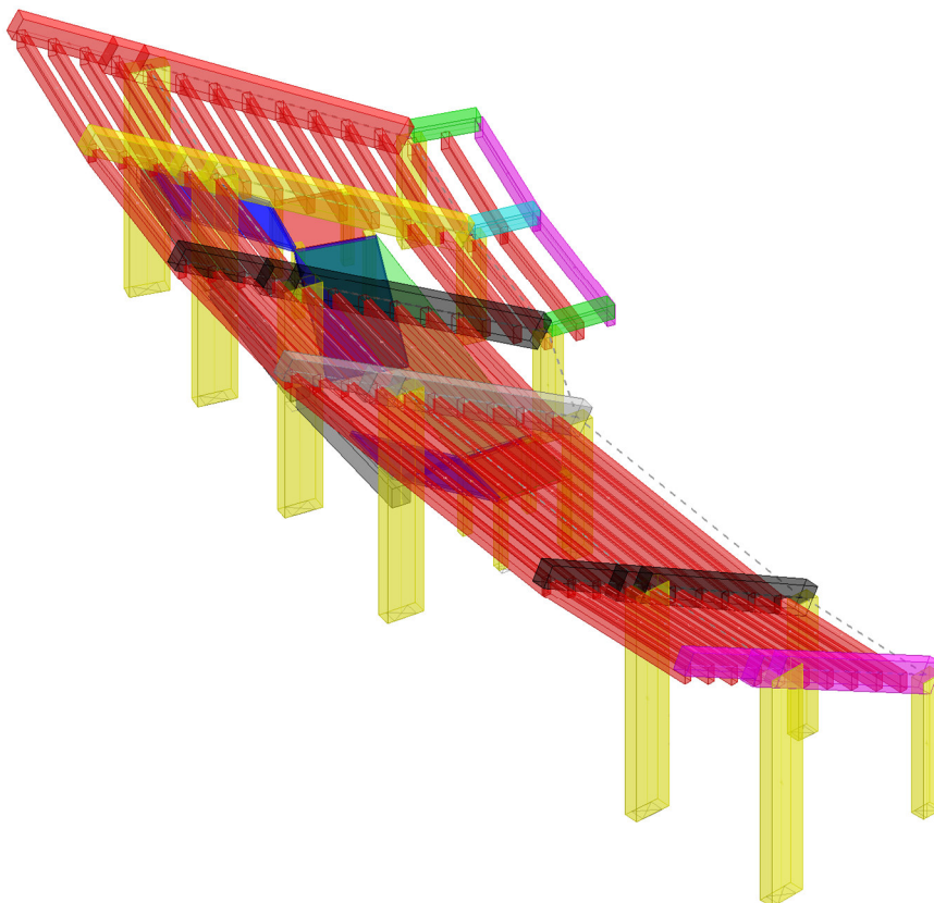
Figura 6.17 – Vista estrusa modello Corpo B-1
