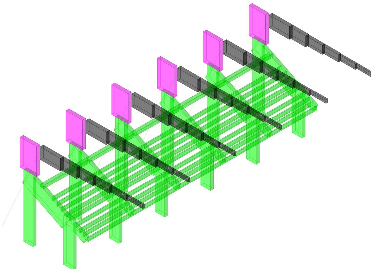
Figura 7.17 – Verifiche SLV Corpo E-2
