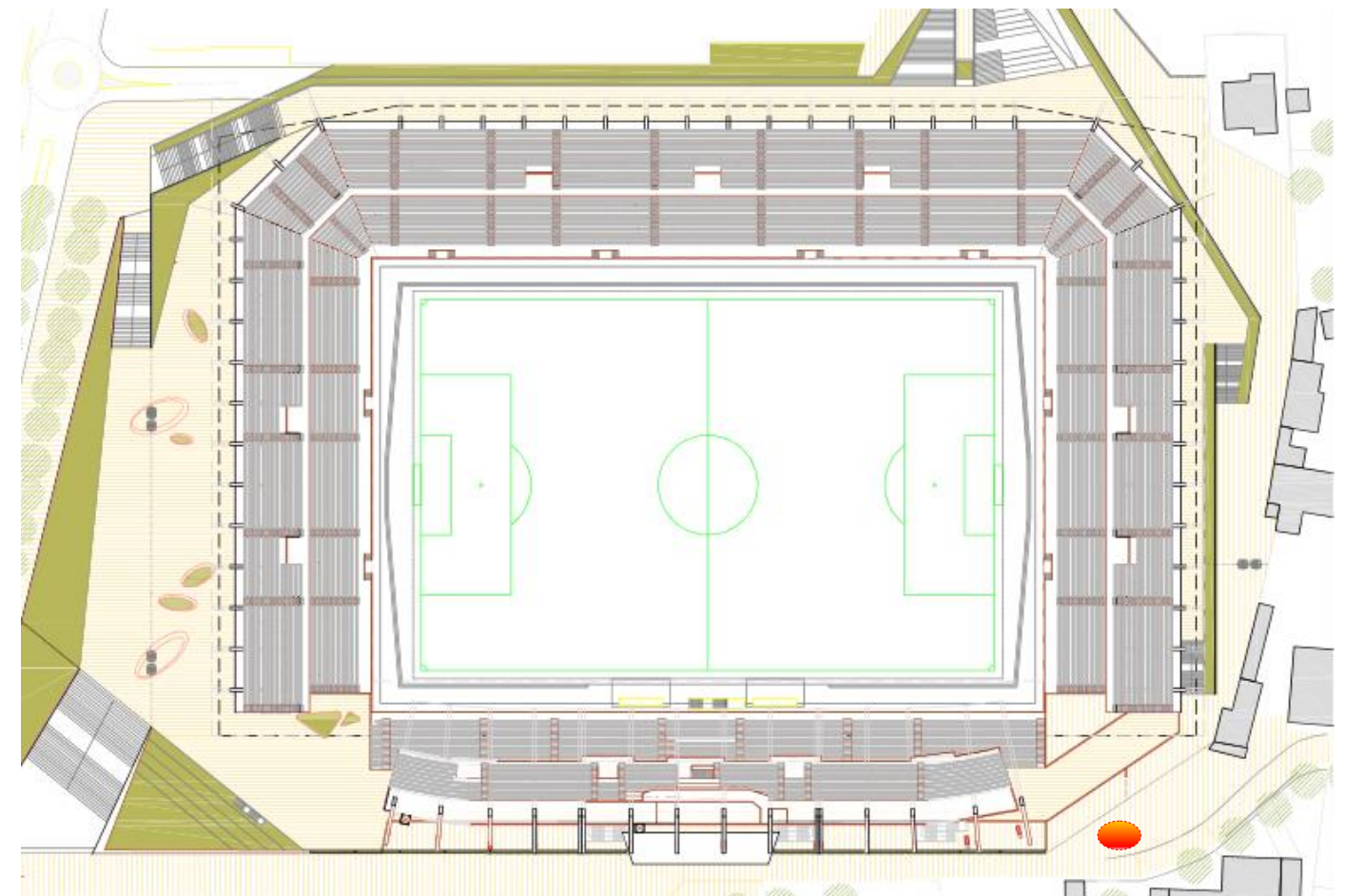
SOTTOSTAZIONE ELETTRICA MT/BT Posizione della sottostazione
