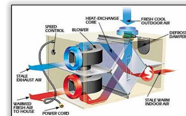
RECUPERATORI DI CALORE Migliora l'efficienza energetica
