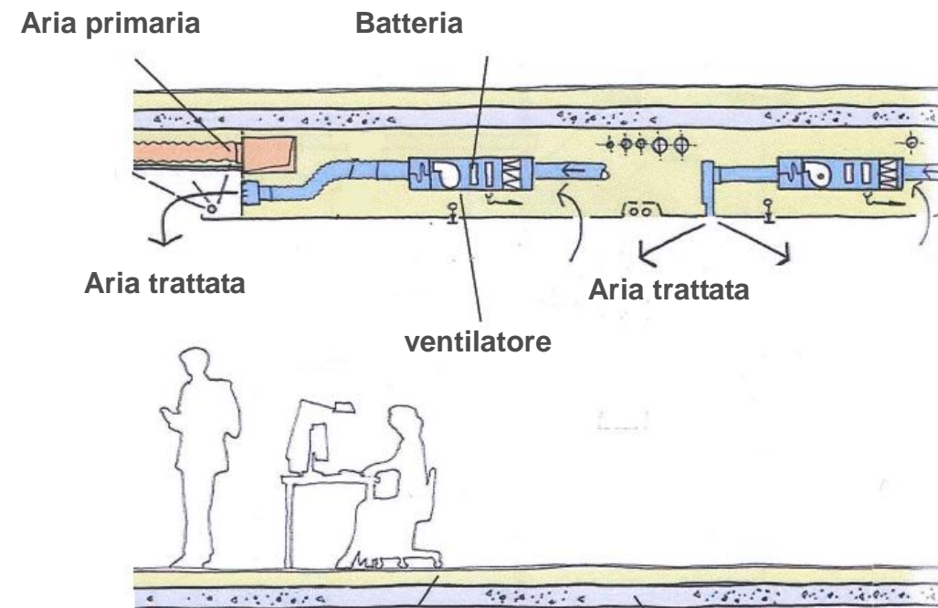
SEZIONE DEL SOFFITTO
