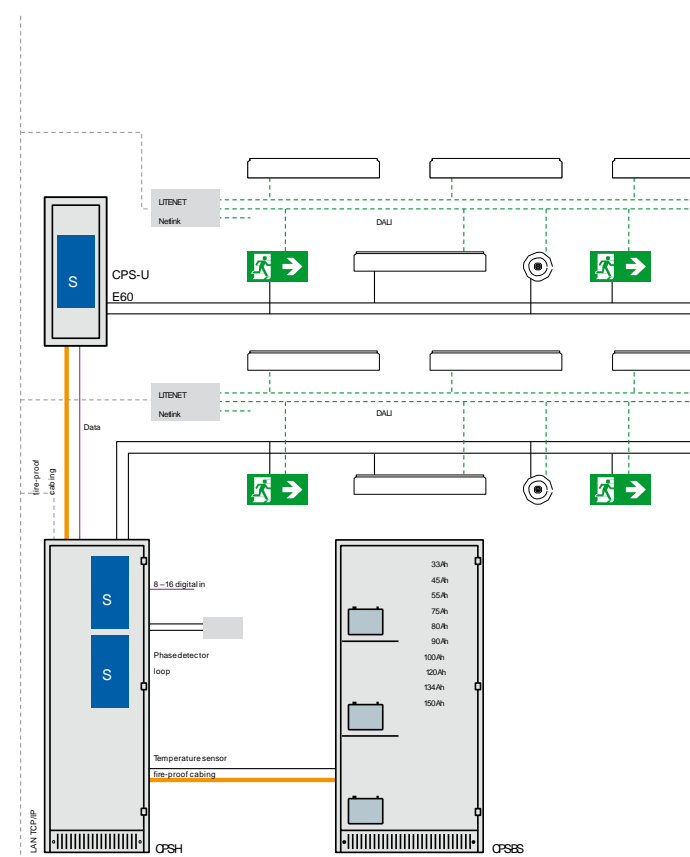
SISTEMA DI ILLUMINAZIONE DI EMERGENZA
