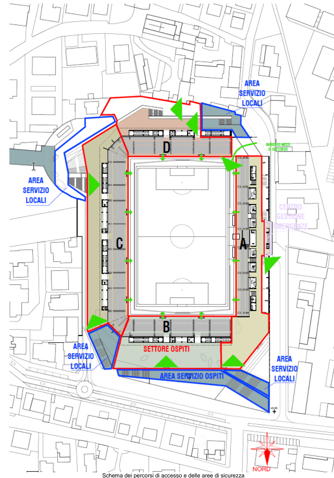
Schema dei percorsi di accesso e delle aree di sicurezza
