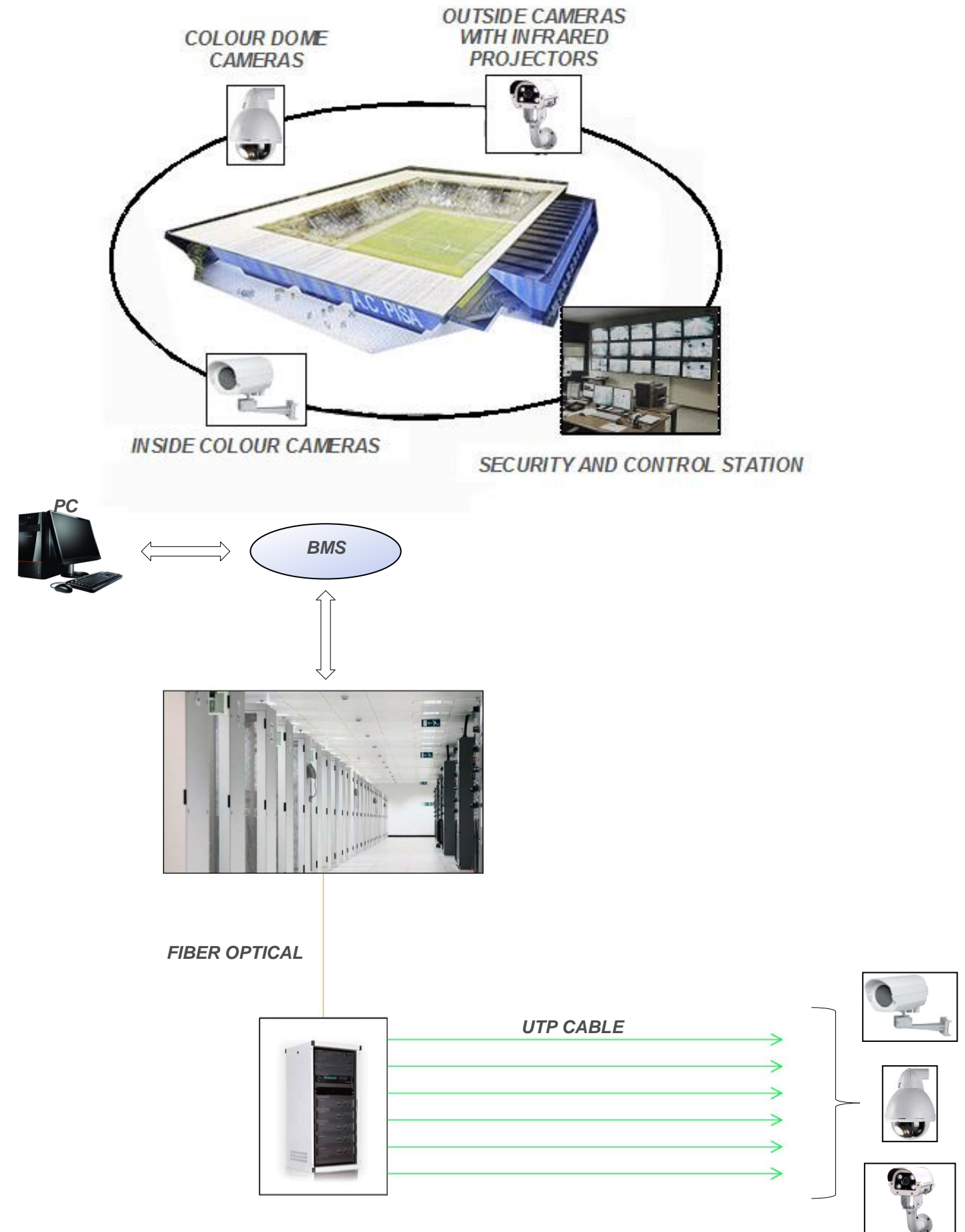
Sistema di videosorveglianza
